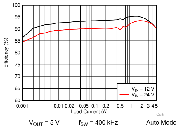
图 8-4. LM76005 Efficiency
