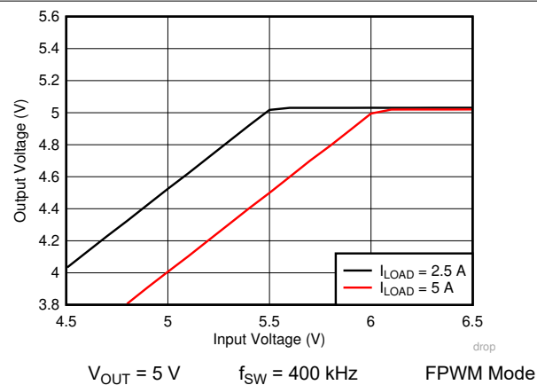
图 8-6. LM76005 Voltage Dropout
