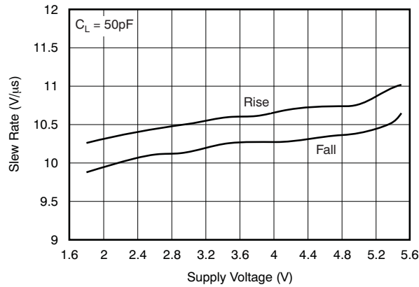
图 25. 压摆率与电源电压间的关系
