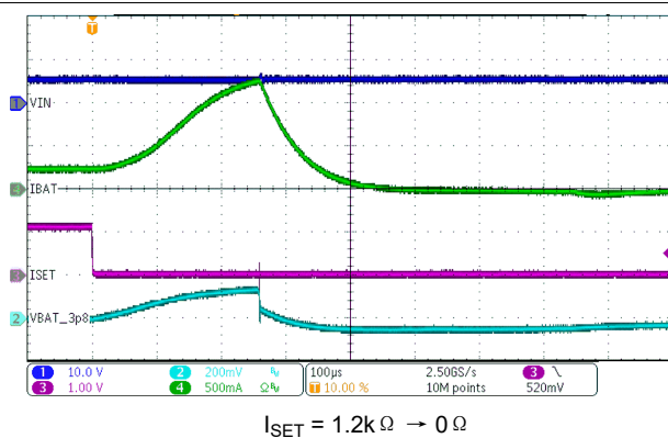
图 8-10. ISET 短路响应
