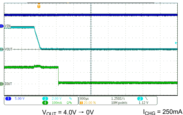
图 8-9. OUT 短路响应
