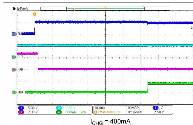
图 8-2. 通过超级电容器上电
