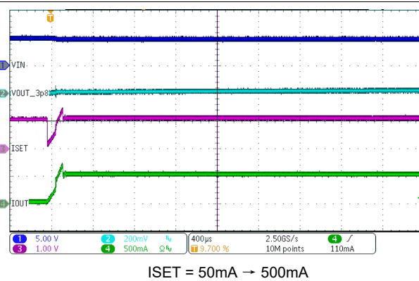
图 8-11. ISET 更改响应
