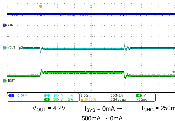
图 8-8. OUT 瞬态响应
