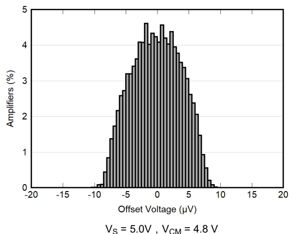
图 6-2. 失调电压分布图
