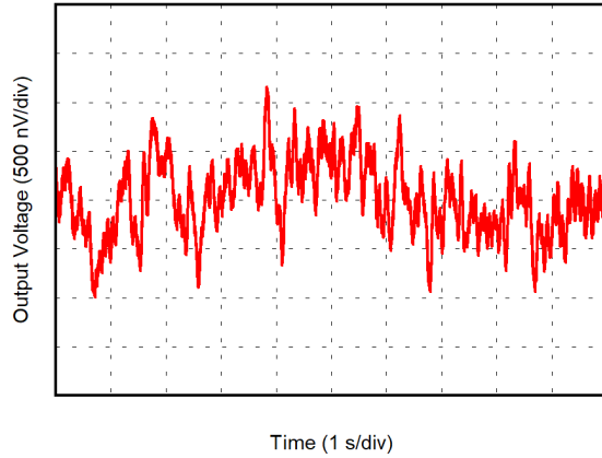
图 6-25. 0.1Hz 至 10Hz 噪声
