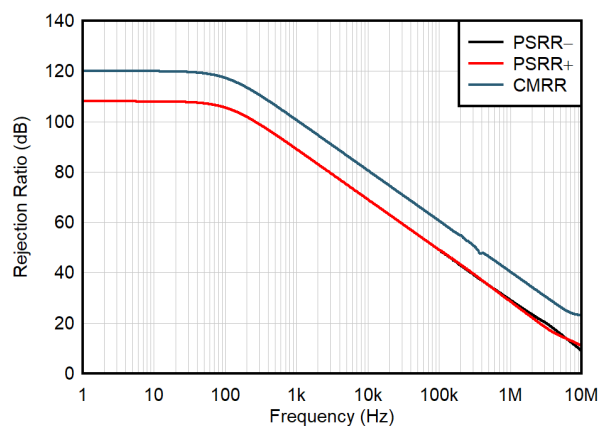
图 6-19. CMRR 和 PSRR 与频率间的关系
