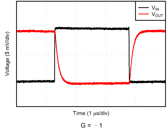
图 6-36. 小信号阶跃响应 (10mV 阶跃)
