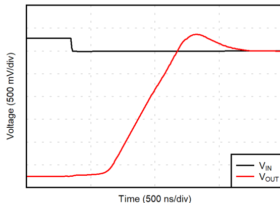
图 6-34. 负过载恢复
