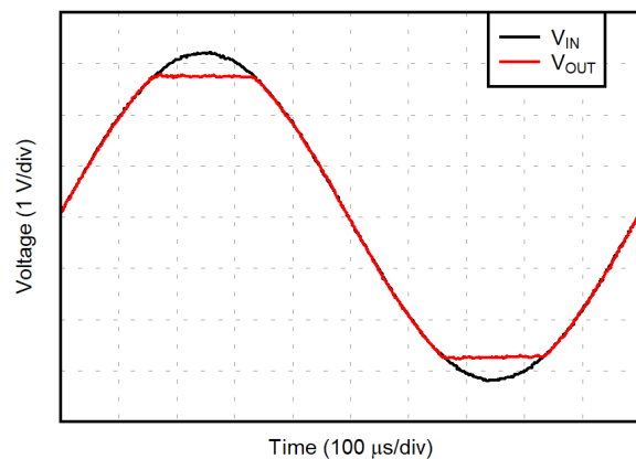
图 6-32. 无相位反转
