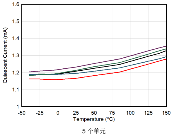
图 6-27. 静态电流与温度间的关系
