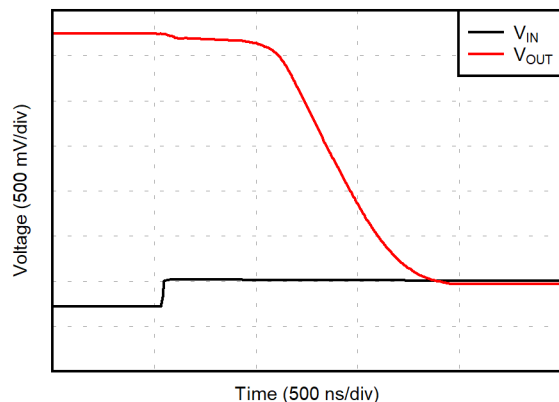
图 6-33. 正过载恢复
