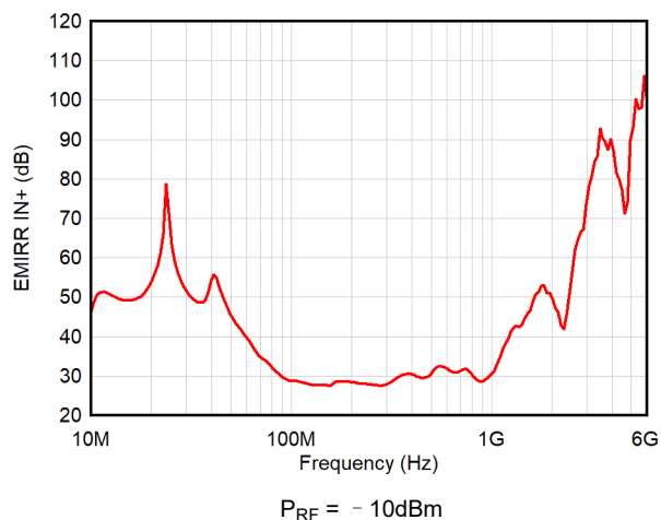
图 6-40. EMIRR 与频率之间的关系
