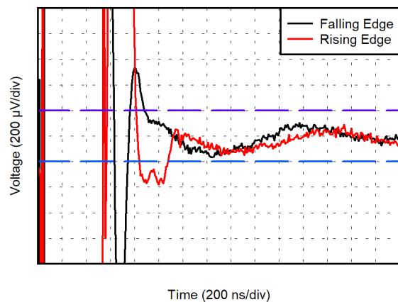
图 6-39. 建立时间
