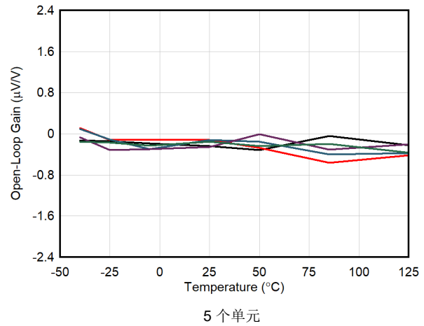
图 6-28. 开环增益与温度间的关系
