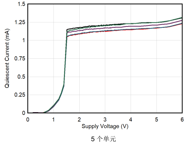
图 6-26. 静态电流与电源电压间的关系
