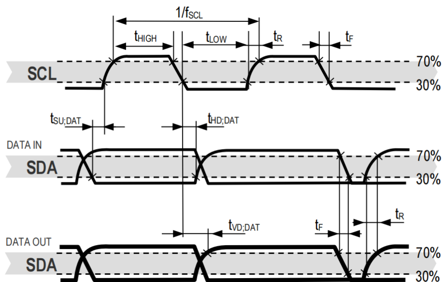
图 6 数字 PAD 的输入输出时序
