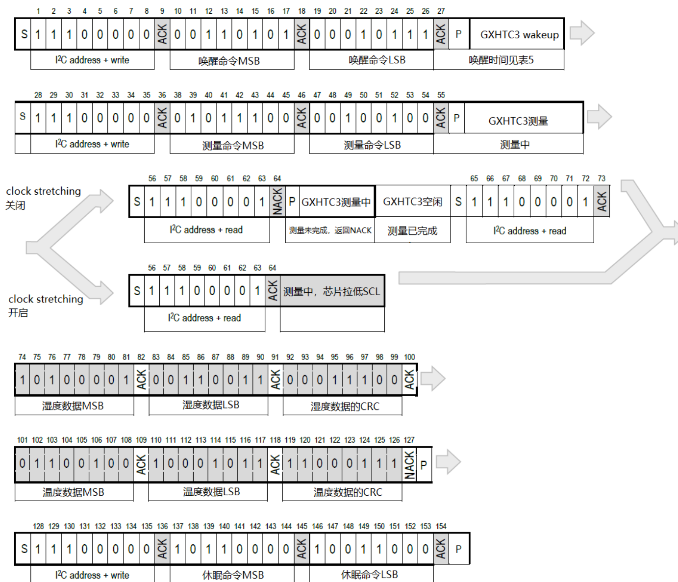
图 8 唤醒传感器、开始温湿度测量、温湿度转换和休眠命令执行顺序示意图
