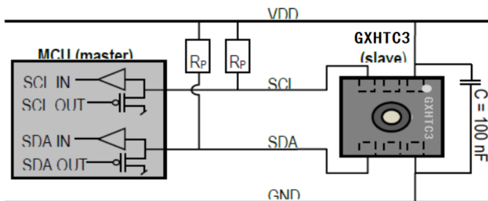
图 7 GXHTC3 的典型应用电路 (包括上拉电阻和去耦电容)。
