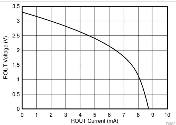
图 5-2. 接收器 VOH 与负载电流间的关系
