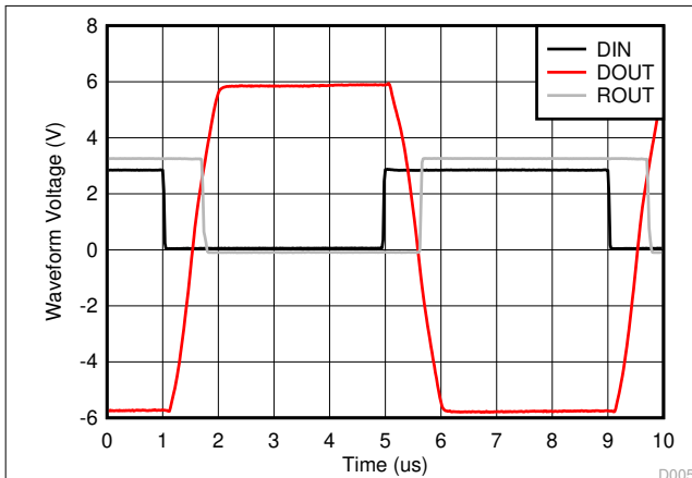
图 8-2. V_{CC} = 3.3V 、数据速率 250kbit/s 时的环回波形
