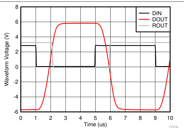
图 8-3. 1nF 负载、 V_{CC} = 3.3V 、数据速率 250kbit/s 时的环回波形
