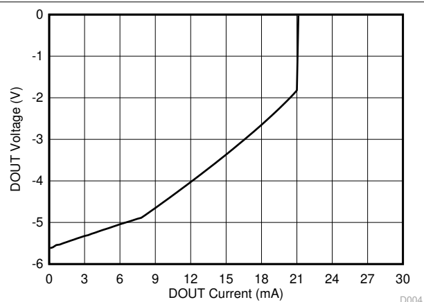
图 5-4. 驱动器 VOL 与负载电流间的关系
