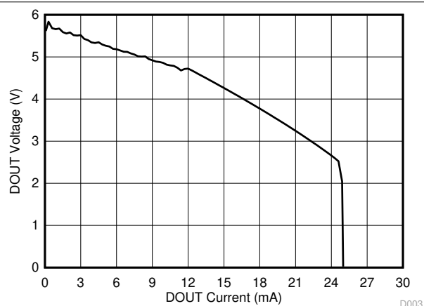
图 5-3. 驱动器 VOH 与负载电流间的关系
