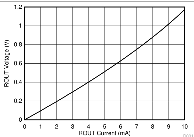
图 5-1. 接收器 VOL 与负载电流间的关系
