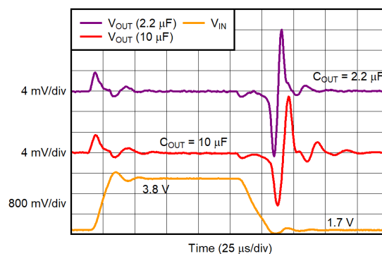
图 7-4. V_{IN} Line Transient
