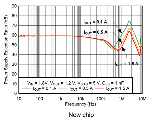
图 5-16. V_{BIAS} PSRR vs Frequency
