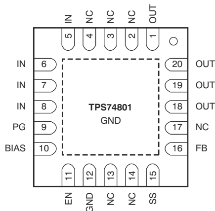
图 4-2. RGW Package, 20-Pin VQFN (Top View)
