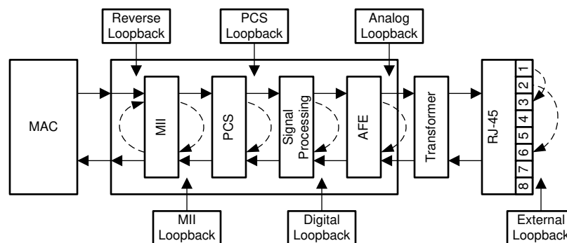
图 7-11. Loopbacks
