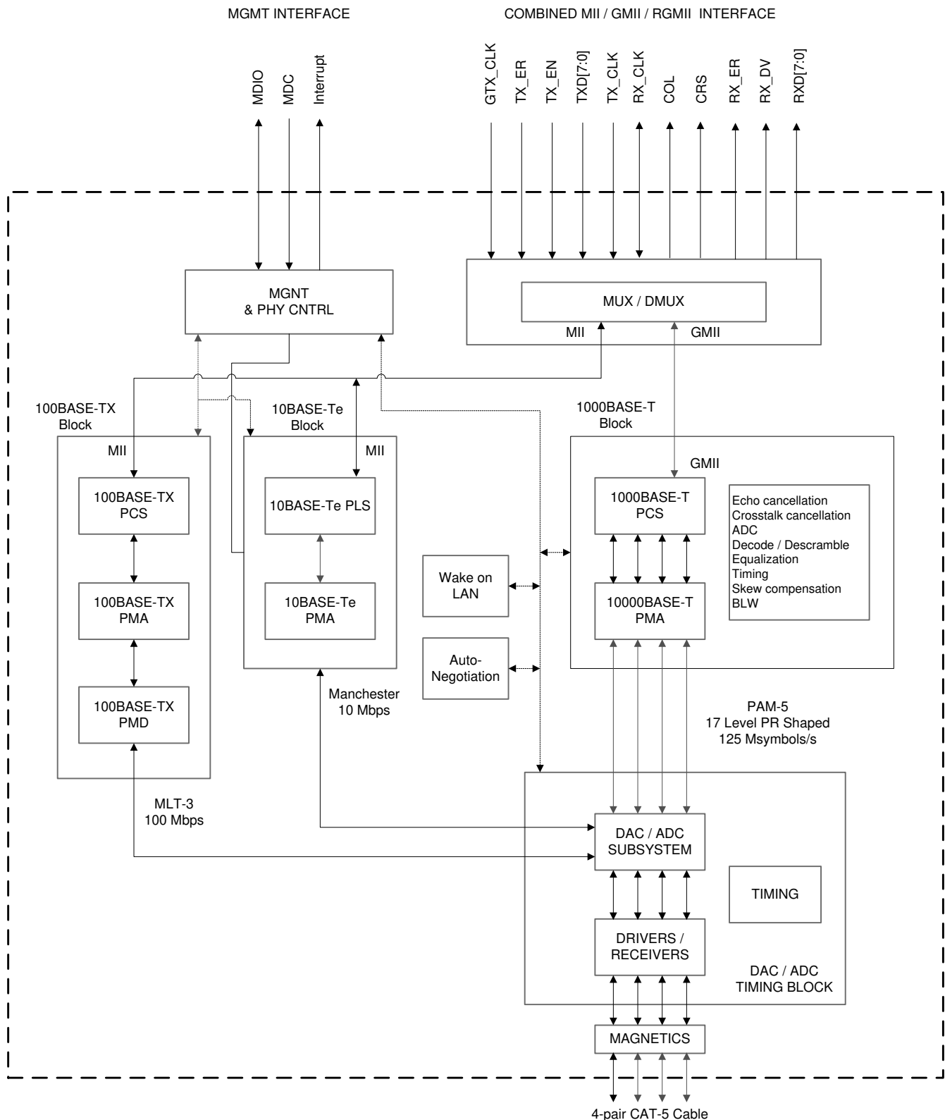
图 7-1. DP83867IRPAP
