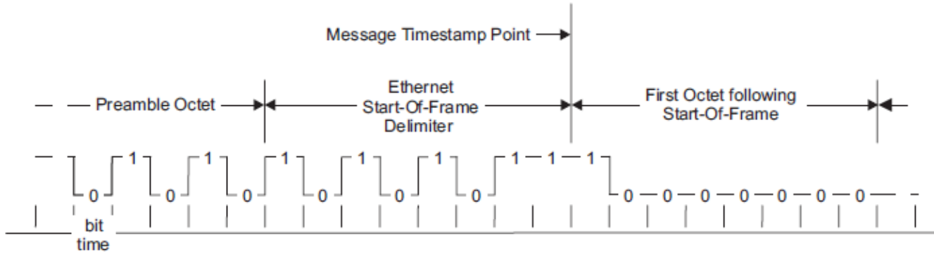
图 7-4. IEEE 1588 Message Timestamp Point
