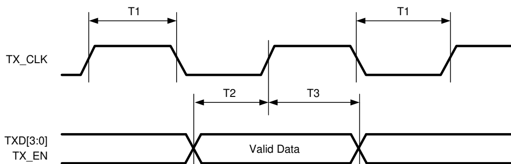
图 6-8. 100Mbps MII Transmit Timing
