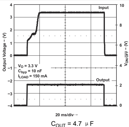
图 8-23. Turn-On Time
