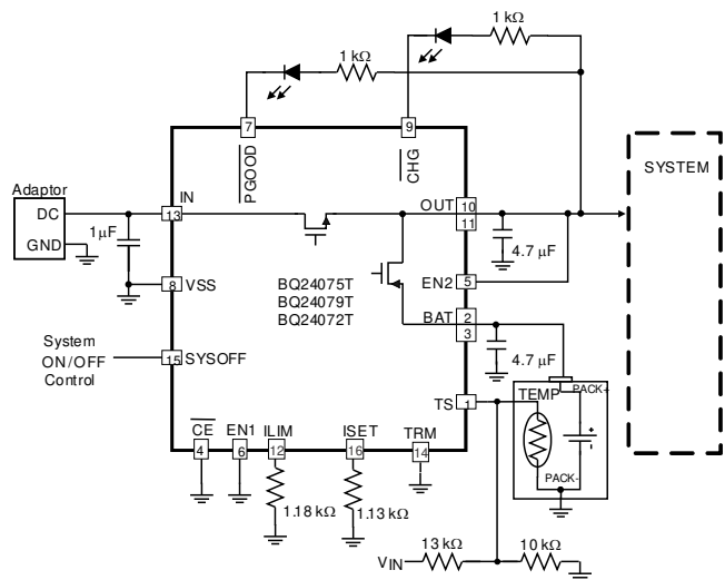
简化电路
