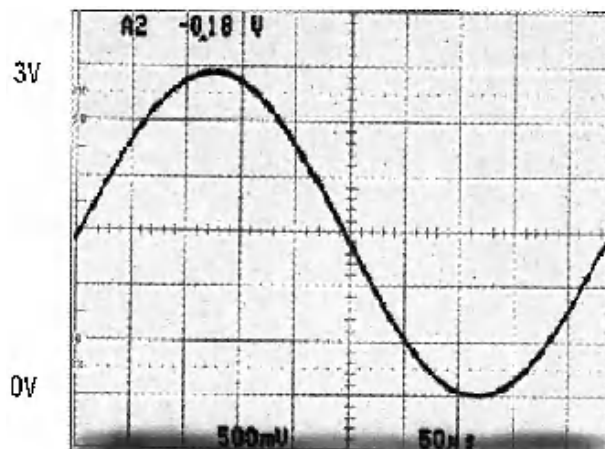
图 7-16. 轨到轨输出
