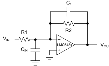
图 7-12. 抵消输入电容的影响
