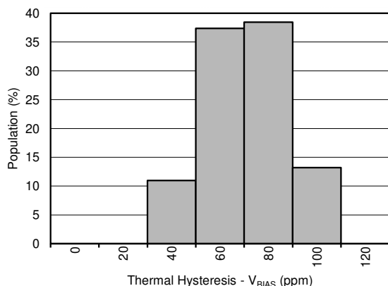
图 7-39. Thermal Hysteresis Distribution ( V_{BIAS} )
