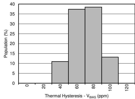
图 8-6. Thermal Hysteresis Distribution (V BIAS )
