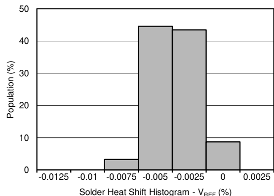
图 7-8. Solder Heat Shift Distribution ( V_{REF} )
