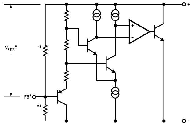
方框图
