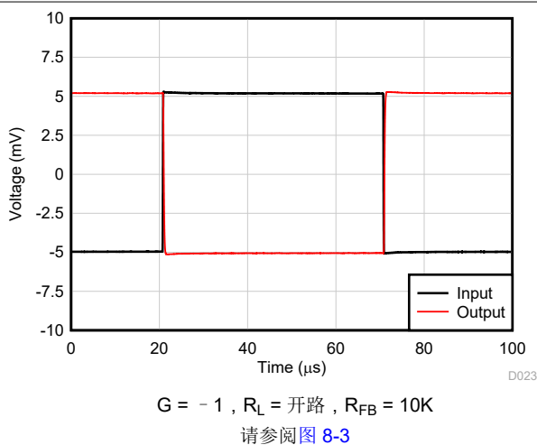
图 7-30. 小信号阶跃响应, G = -1
