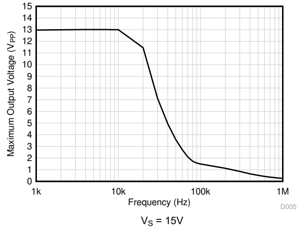
图 7-36. 最大输出电压与频率间的关系
