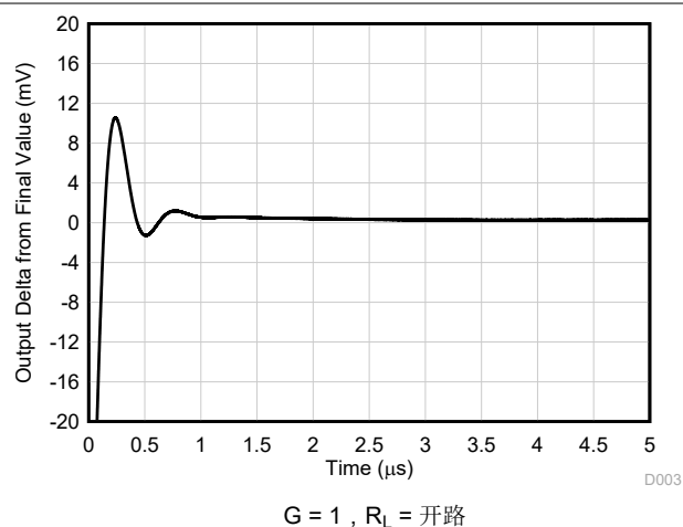
图 7-31. 大信号阶跃响应 (上升)
