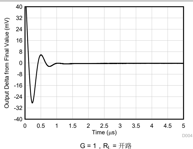
图 7-32. 大信号阶跃响应 (下降)
