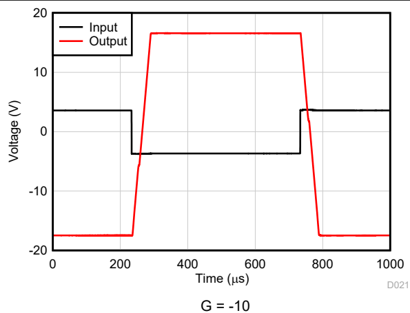
图 7-28. 过载恢复
