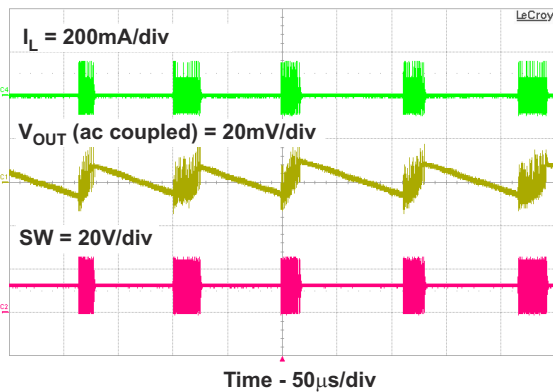
图 8-7. Pulse Skipping
