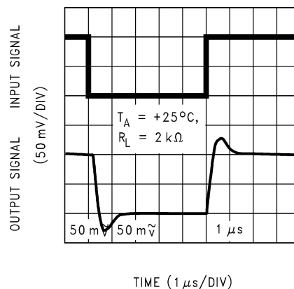
图 5-32. 同相小信号脉冲响应
