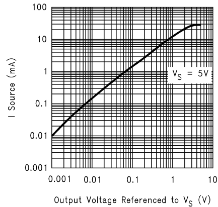
图 5-4. 拉电流与输出电压之间的关系
