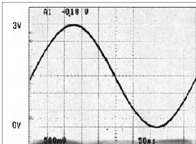
图 7-15. 轨到轨输入
