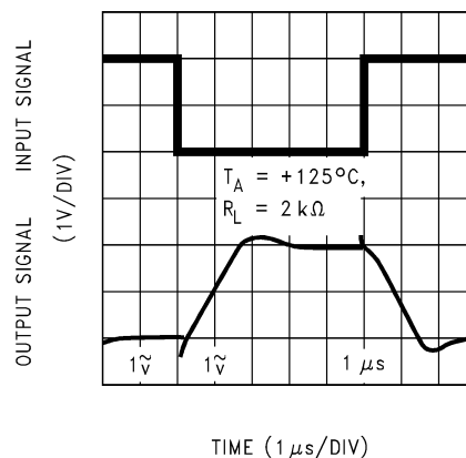
图 5-34. 反相大信号脉冲响应
