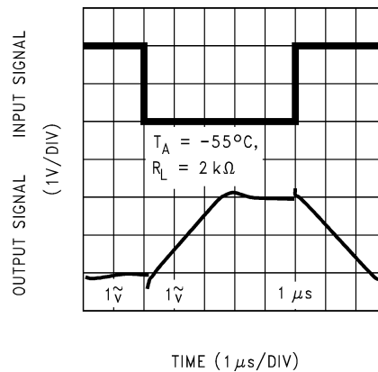
图 5-36. 反相大信号脉冲响应
