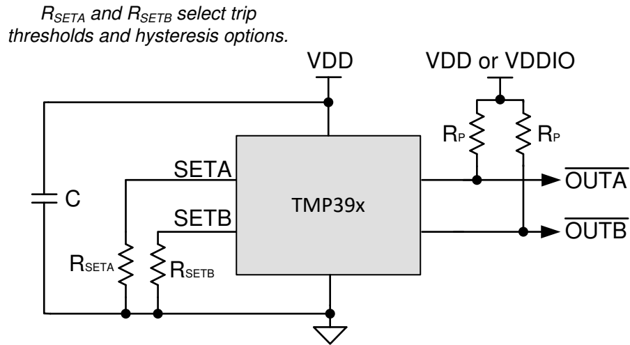
图 7-1. 简化原理图
