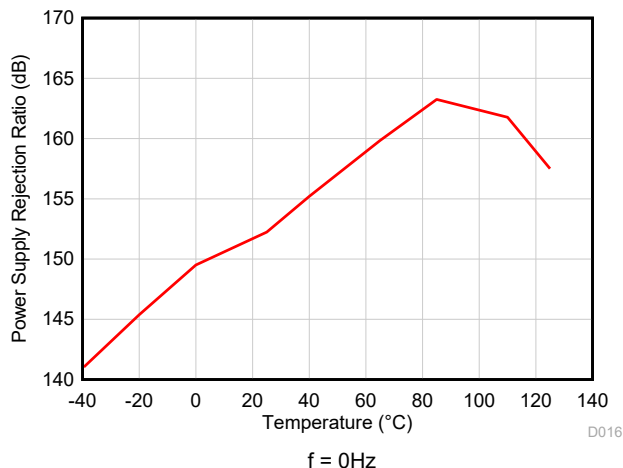
图 6-18. PSRR 与温度之间的关系 (dB)
