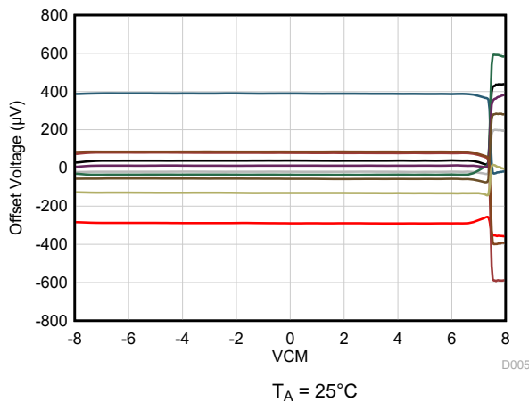
图 6-5. 失调电压与共模电压之间的关系
