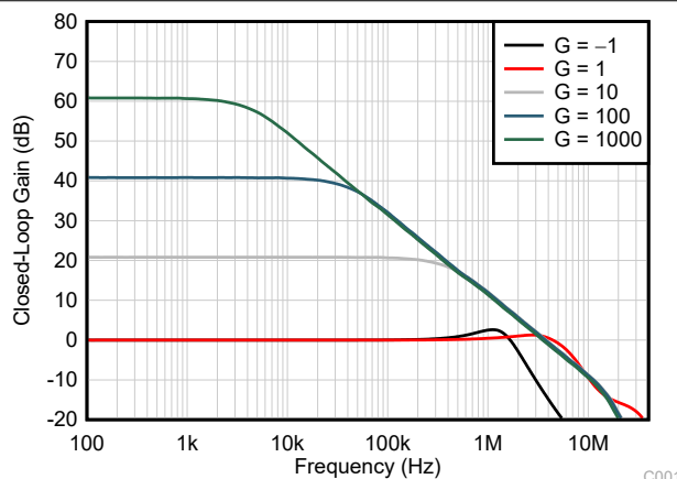
图 6-11. 闭环增益与频率之间的关系
