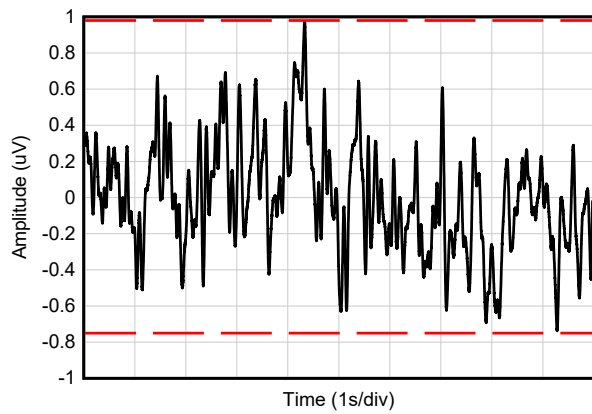
图 6-19. 0.1Hz 至 10Hz 噪声
