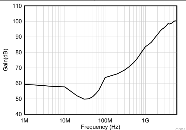
图 6-41. EMIRR (电磁干扰抑制比) 与频率之间的关系
