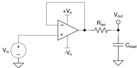
图 7-5. 使用 TLV9151 扩展容性负载驱动
