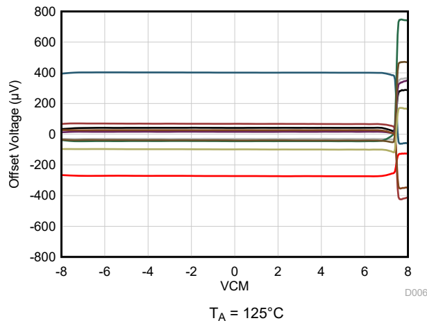
图 6-7. 失调电压与共模电压之间的关系
