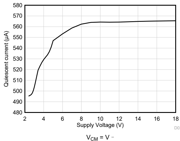
图 6-23. 静态电流与电源电压之间的关系
