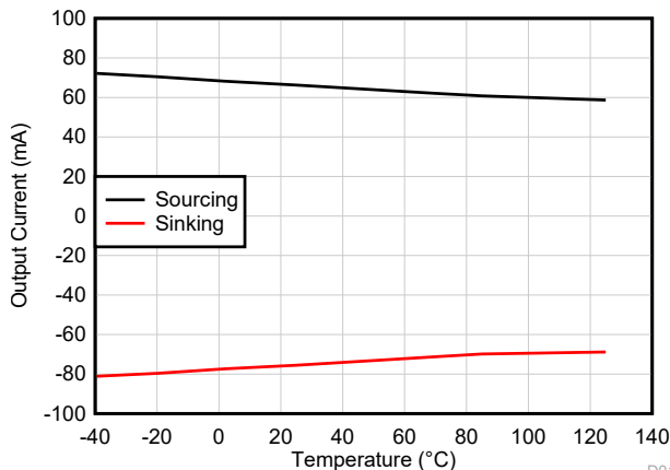
图 6-38. 短路电流与温度之间的关系
