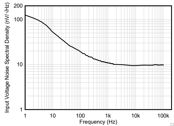
图 6-20. 输入电压噪声频谱密度与频率之间的关系
