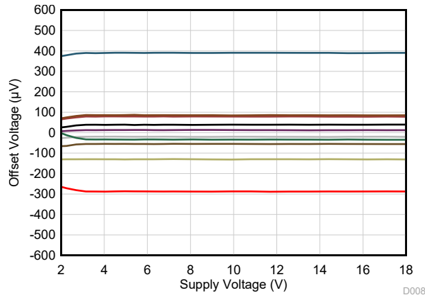
图 6-9. 失调电压与电源之间的关系
