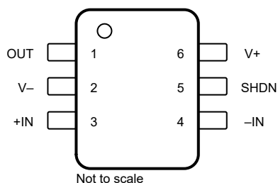
图 5-3. TLV9151S DBV 封装 6 引脚 SOT-23 ( 顶视图 )
