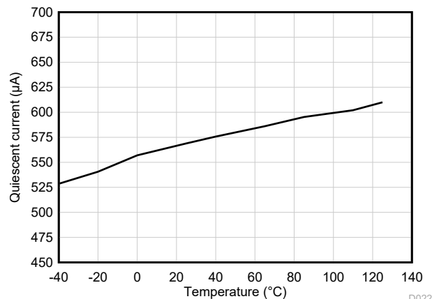
图 6-24. 静态电流与温度之间的关系
