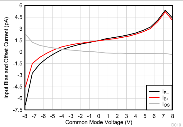
图 6-12. 输入偏置电流与共模电压之间的关系
