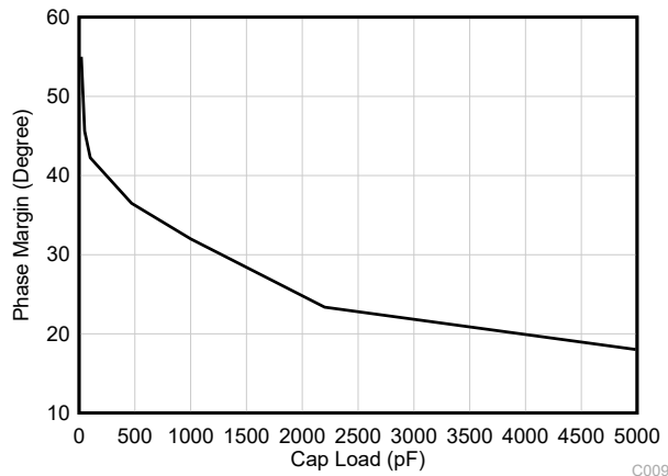
图 6-29. 相位裕度与容性负载之间的关系
