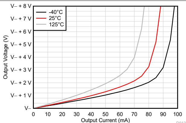
图 6-15. 输出电压摆幅与输出电流 (灌电流) 之间的关系
