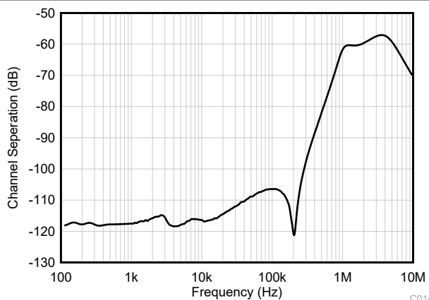
图 6-40. 通道隔离与频率之间的关系
