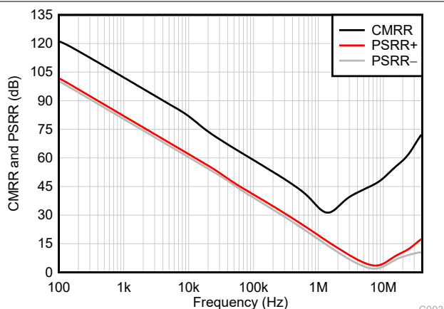
图 6-16. CMRR 和 PSRR 与频率之间的关系
