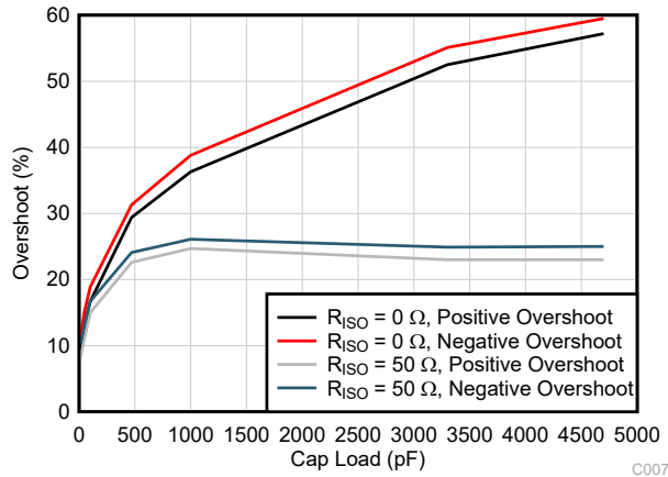
图 6-27. 小信号过冲与容性负载之间的关系
