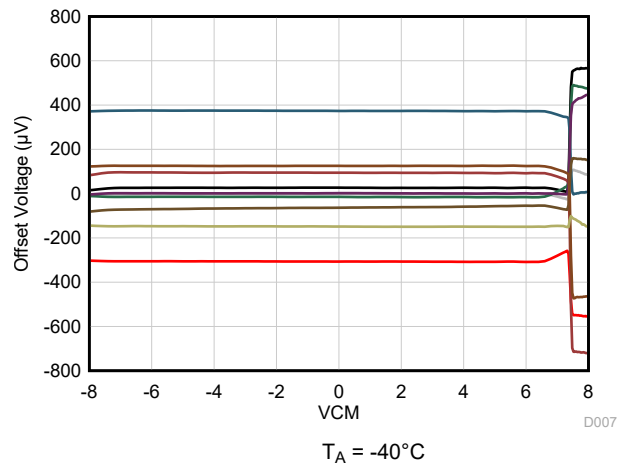
图 6-8. 失调电压与共模电压之间的关系
