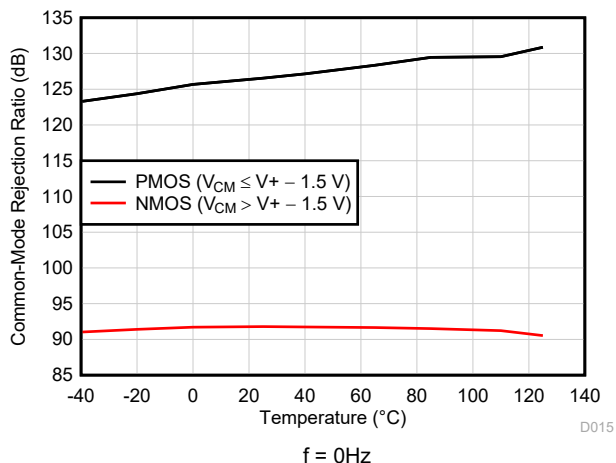
图 6-17. CMRR 与温度之间的关系 (dB)
