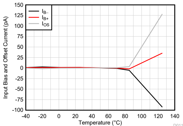
图 6-13. 输入偏置电流与温度之间的关系
