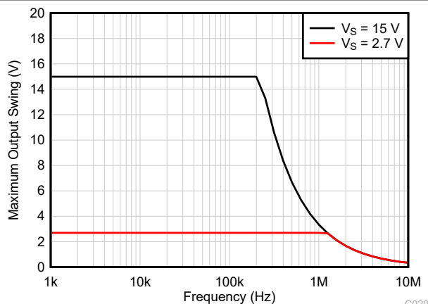
图 6-39. 最大输出电压与频率之间的关系
