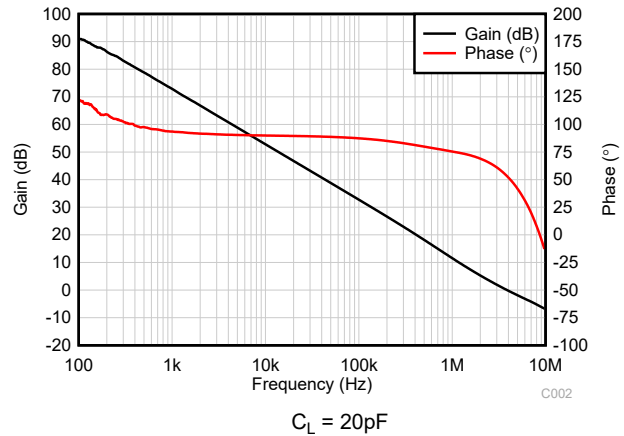
图 6-10. 开环增益和相位与频率之间的关系
