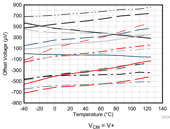
图 6-3. 失调电压与温度之间的关系
