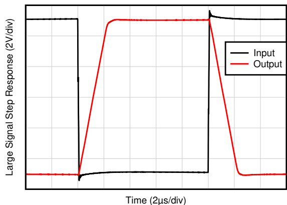
图 6-37. 大信号阶跃响应
