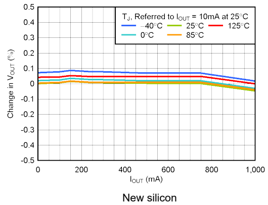
图 5-2. Load Regulation
