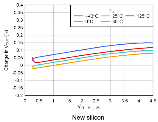
图 5-4. Line Regulation
