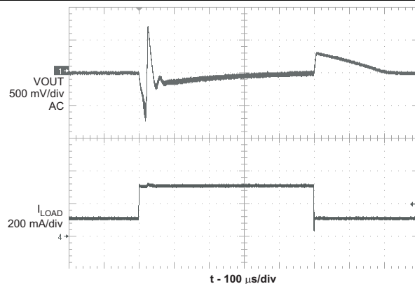
图 13. Load Transient Response
