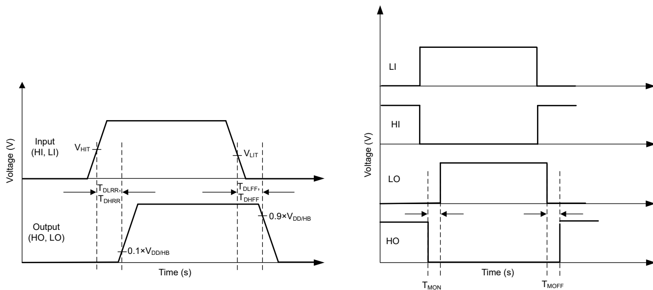
图 5-1. 时序图
