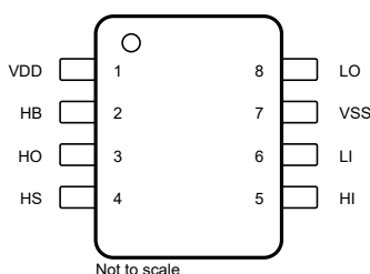
图 4-2. D 封装 8 引脚 SOIC 底视图
