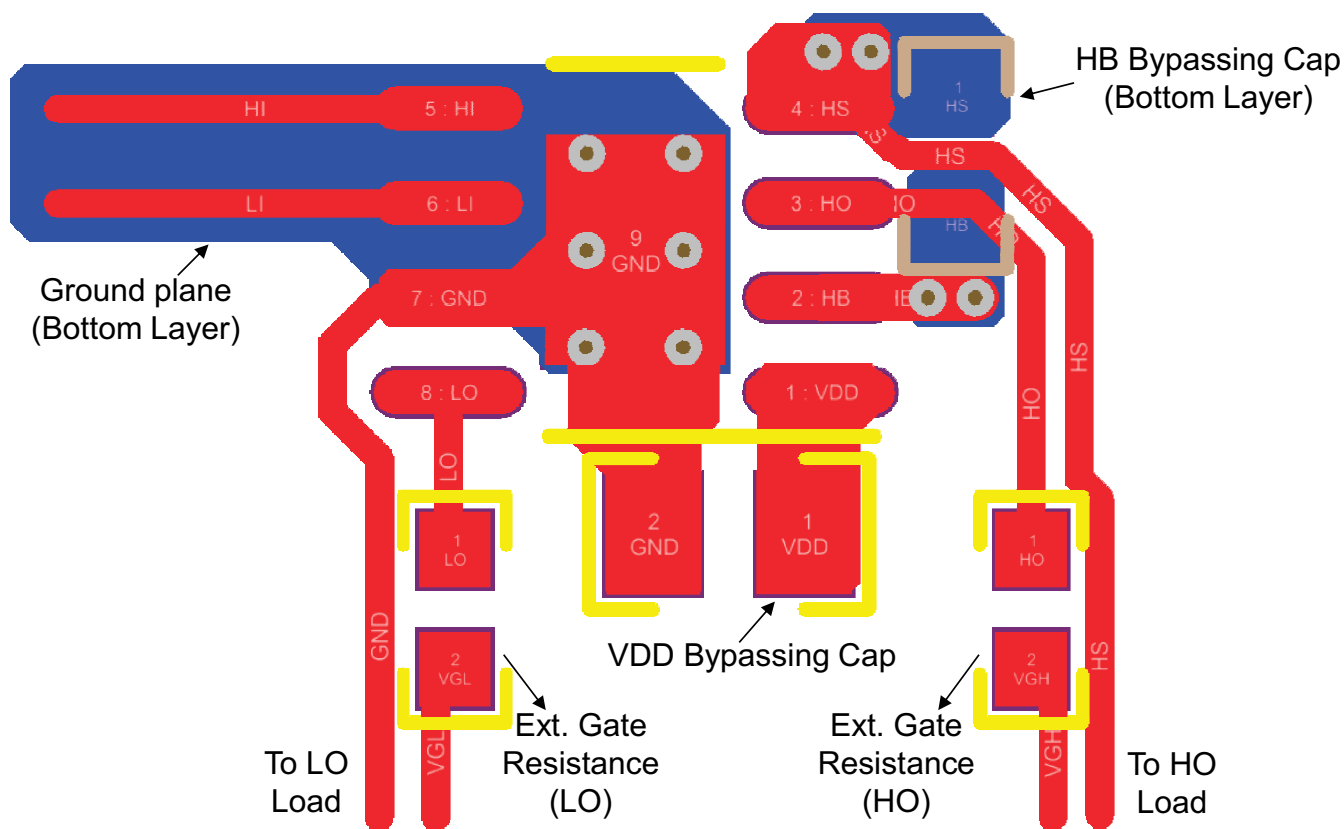
图 9-1. UCC27211A-Q1 PCB 布局示例
