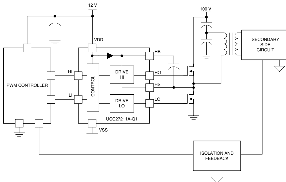
图 7-1. UCC27211A-Q1 典型应用图 1
