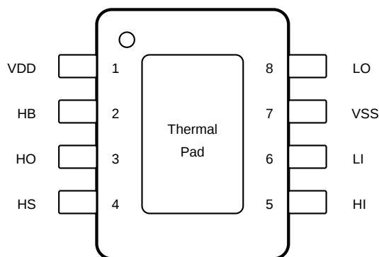
图 4-1. DDA 封装 8 引脚 SO-PowerPAD 顶视图
