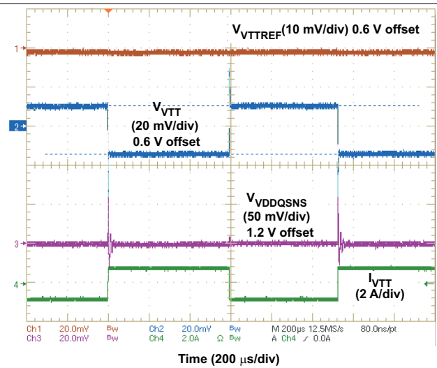
图 16. VTT Load Transient Response (0.6 V)
