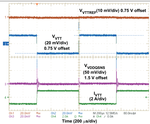
图 14. VTT Load Transient Response (0.75 V)
