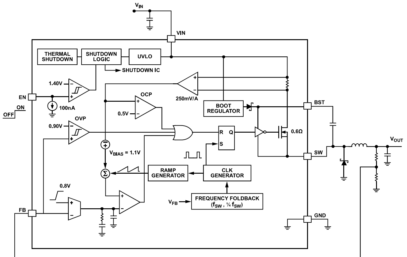
图 4 内部功能框图
