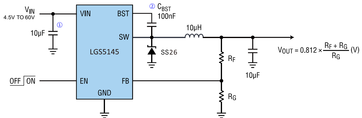
图 5.a DC-DC 降压模式典型应用拓扑
