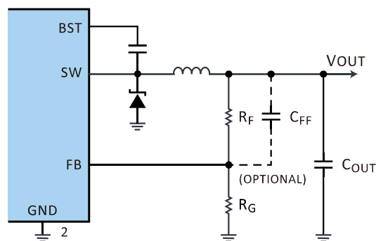
图 6.1 BUCK 恒压模式与 CFF 前置补偿电容
