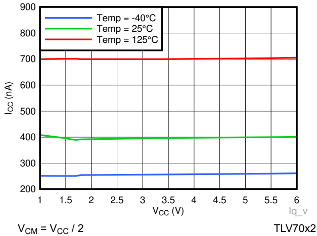
图 6-23. I_{CC} vs V_{CC}
