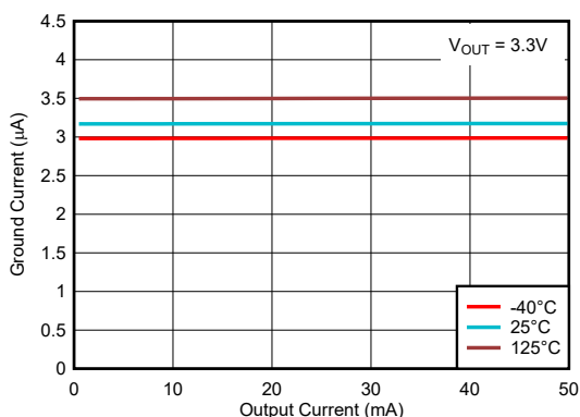
图 3-1. TPS715xx 的静态电流与负载电流 (仅限新芯片)
