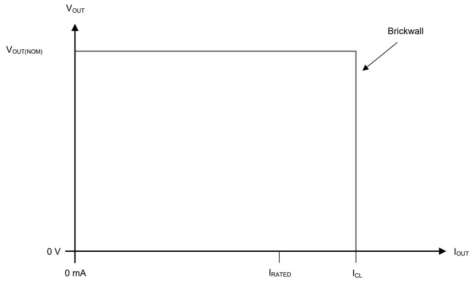
图 7-3. Current Limit
