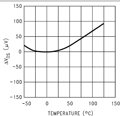
图 5-2. Offset Voltage
