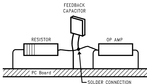
图 6-21. Air Wiring
