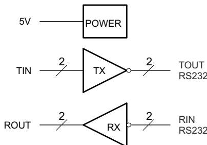
简化原理图
