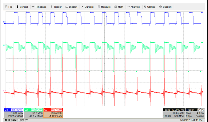
Figure 31. 265-V AC , 3-A Load
