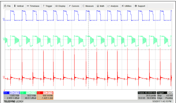
Figure 29. 85-V AC , 3-A Load
