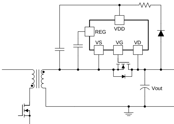
具有高侧 SR 的反激式
