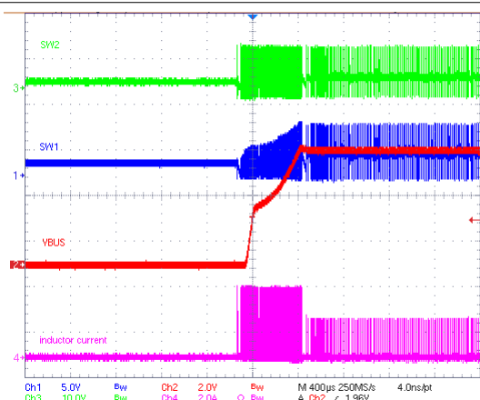
图 10-3. Buck Mode PFM with OOA
