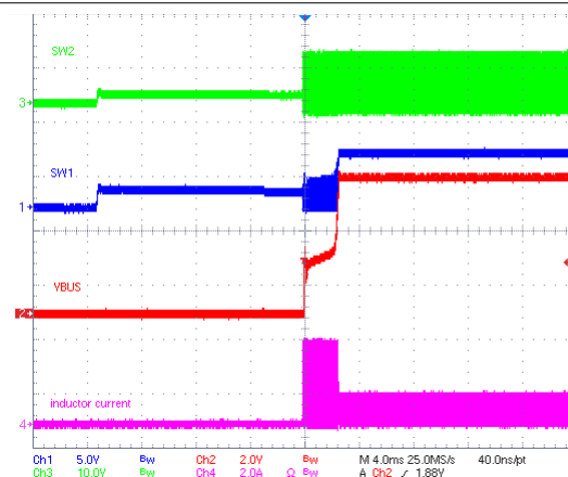
图 10-4. Buck Mode PFM without OOA
