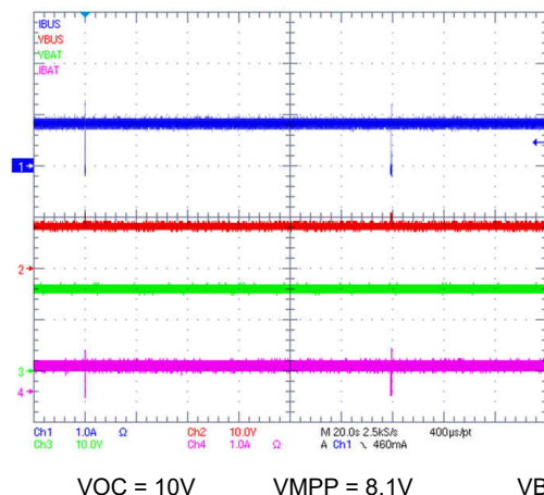
图 10-10. MPPT Operation
