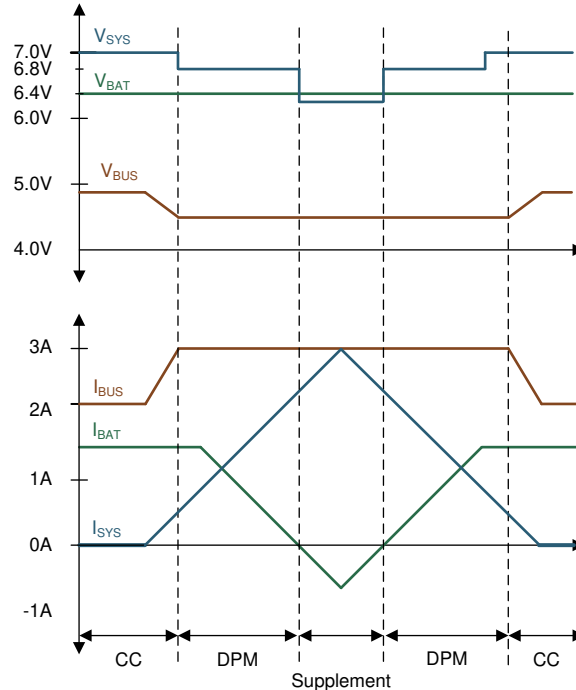
图 9-8. DPM Response
