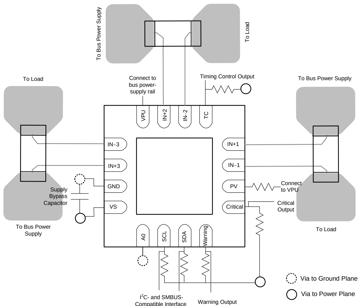
图 55. Layout Example
