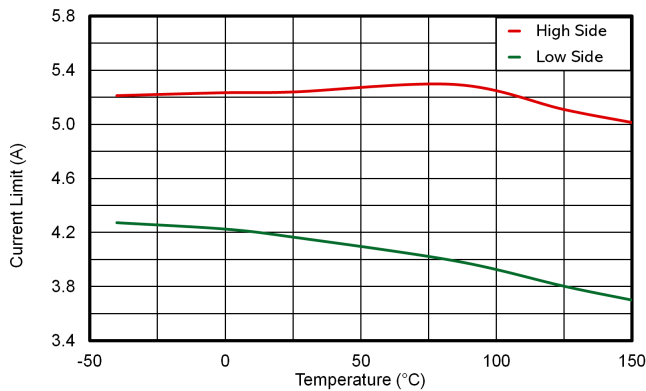
图 6-15. LMR51635 HS 和 LS 电流限制与温度间的关系
