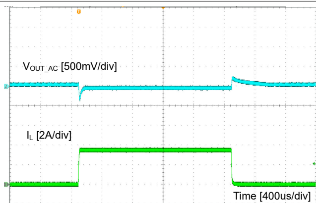
图 8-7. 负载瞬态
