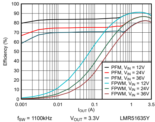
图 6-3. 效率与负载电流间的关系 (3.3V)
