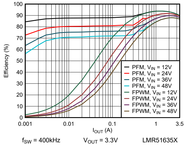
图 6-1. 效率与负载电流间的关系 (3.3V)
