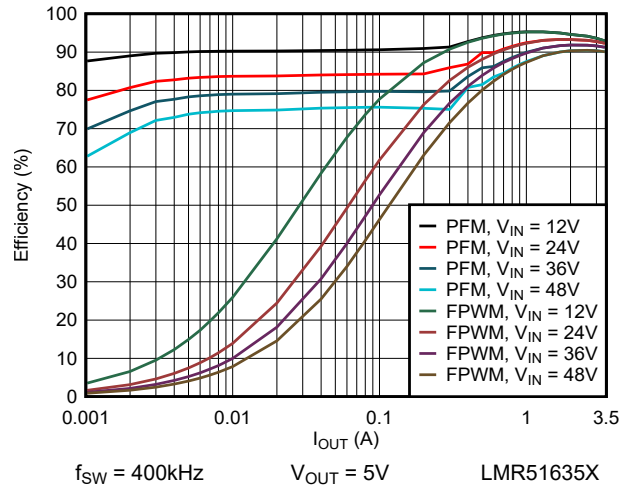
图 6-2. 效率与负载电流间的关系 (5V)
