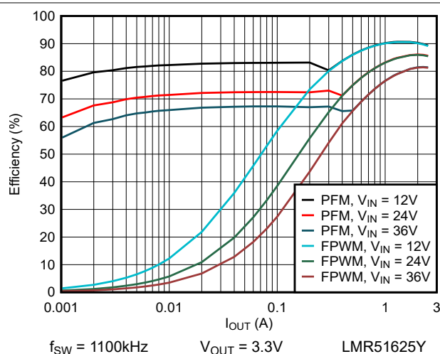
图 6-7. 效率与负载电流间的关系 (3.3V)
