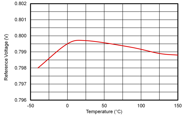
图 6-12. 基准电压与温度间的关系
