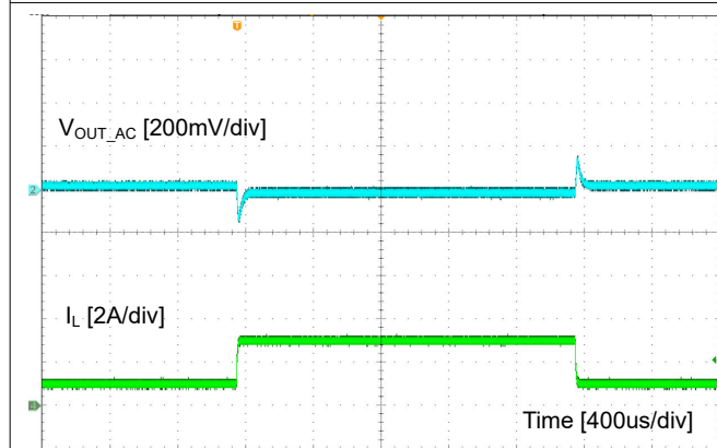
图 8-6. 负载瞬态
