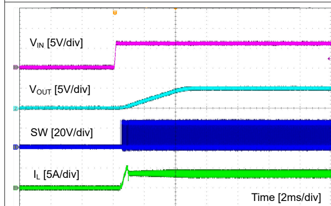
图 8-4. 由 V_{IN} 启动
