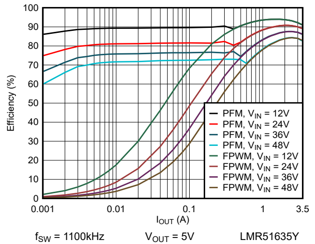
图 6-4. 效率与负载电流间的关系 (5V)
