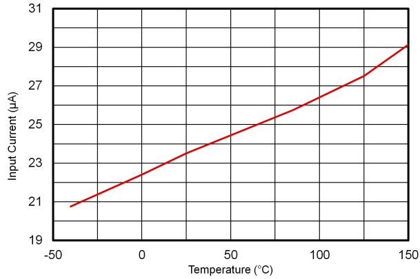
图 6-11. I_Q 与温度间的关系
