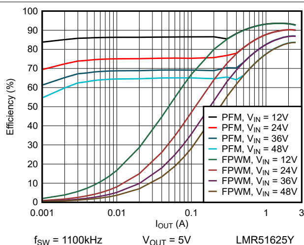
图 6-8. 效率与负载电流间的关系 (5V)
