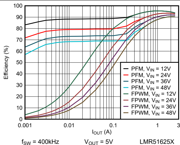
图 6-6. 效率与负载电流间的关系 (5V)
