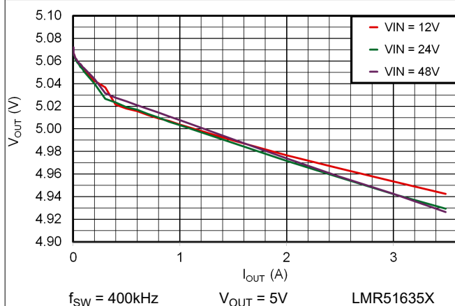
图 6-9. 线性和负载调整率
