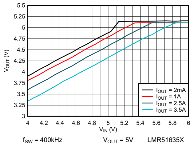
图 6-10. 5V 压降
