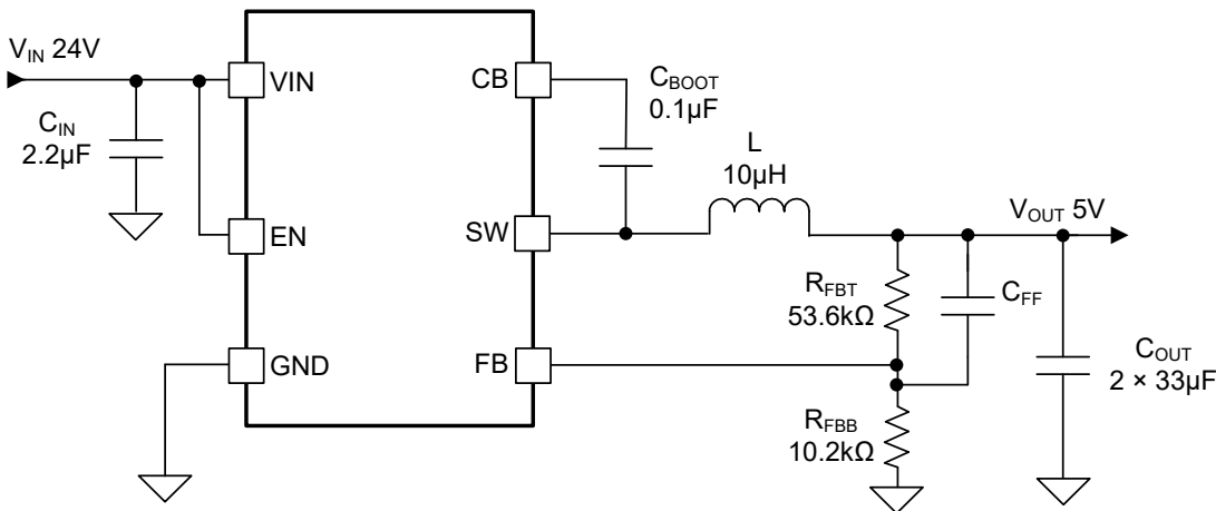
图 8-1. 应用电路
