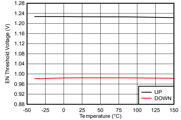
图 6-14. 精密使能阈值
