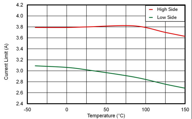
图 6-16. LMR51625 HS 和 LS 电流限制与温度间的关系
