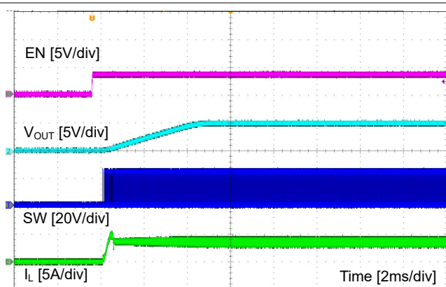
图 8-5. 由 EN 启动
