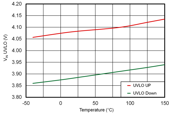
图 6-13. V_{IN} UVLO 与温度间的关系
