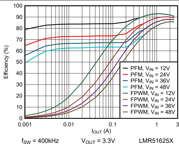
图 6-5. 效率与负载电流间的关系 (3.3V)
