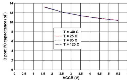
图 5-3. B 端口 I/O 引脚的电容 ( C_{iO} ) 与 V_{CCA} = 3.3\text{V} 时的电源 ( V_{CCB} ) 间的关系 (RUT 封装)
