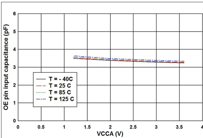
图 5-1. OE 引脚的输入电容 ( C_i ) 与 V_{CCB} = 3.3\text{V} 时的电源电压 ( V_{CCA} ) 间的关系 (RUT 封装)
