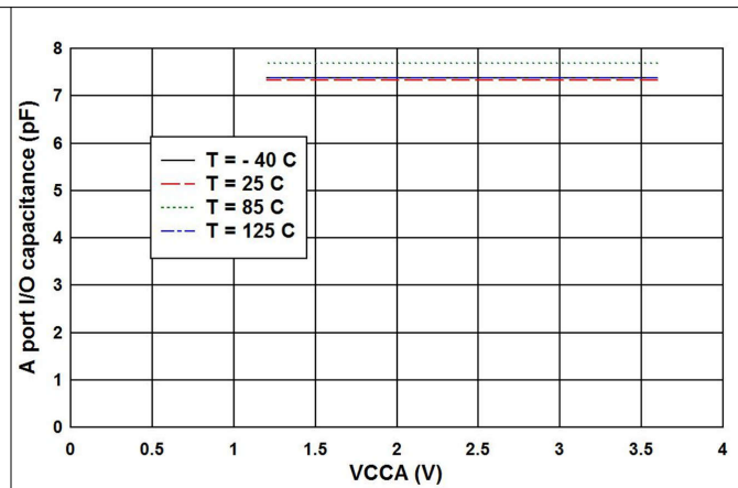
图 5-2. A 端口 I/O 引脚的电容 ( C_{iO} ) 与 V_{CCB} = 3.3\text{V} 时的电源 ( V_{CCA} ) 间的关系 (RUT 封装)
