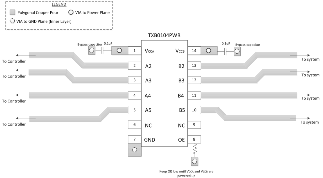
图 10-1. 原理图布局示例
