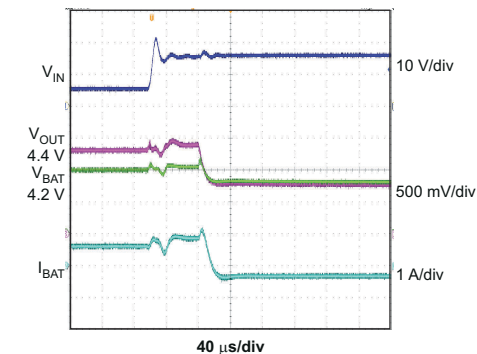
图 10-9. OVP Fault
