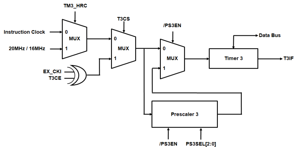
图 24 定时器 3 结构框图
