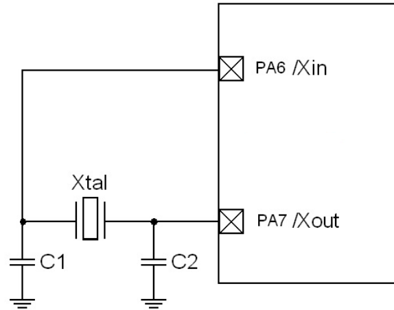
图 35 外部晶体振荡器的硬件连接图
