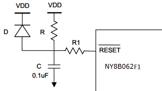
图 38 复位应用框图
