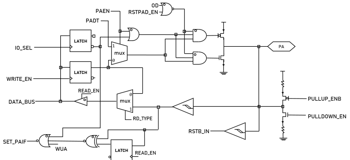
图 8 PA5 引脚结构框图
