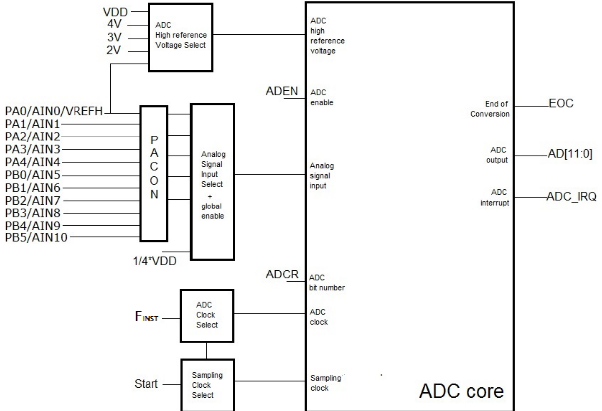
图 33 ADC结构框图
