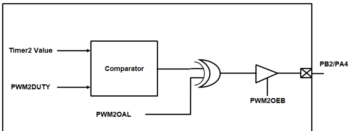
图 22 PWM2 结构框图
