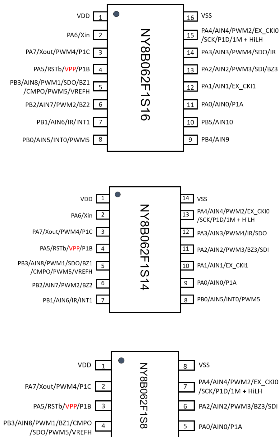
图 1 封装引脚图
