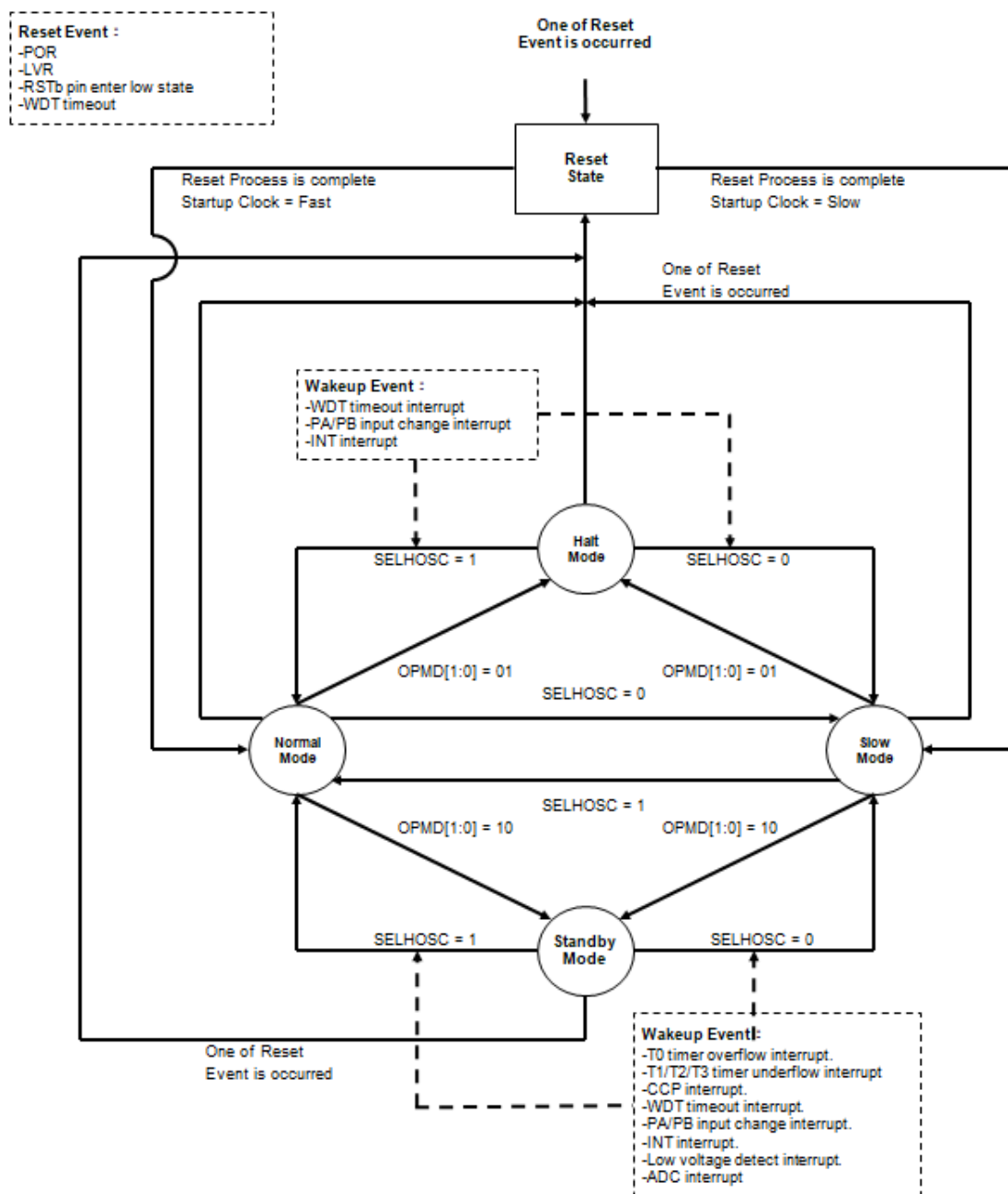
图 36 四种工作模式
