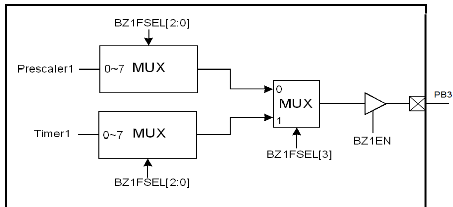
图 19 蜂鸣器 1 结构框图
