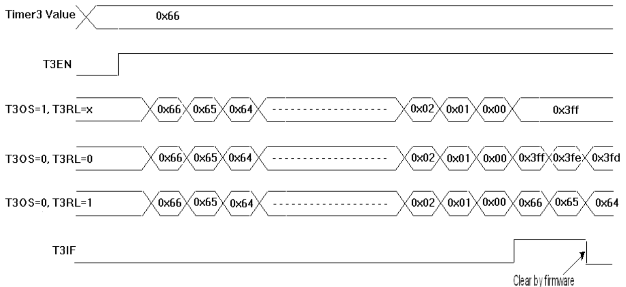
图 25 定时器 3 结构框图
