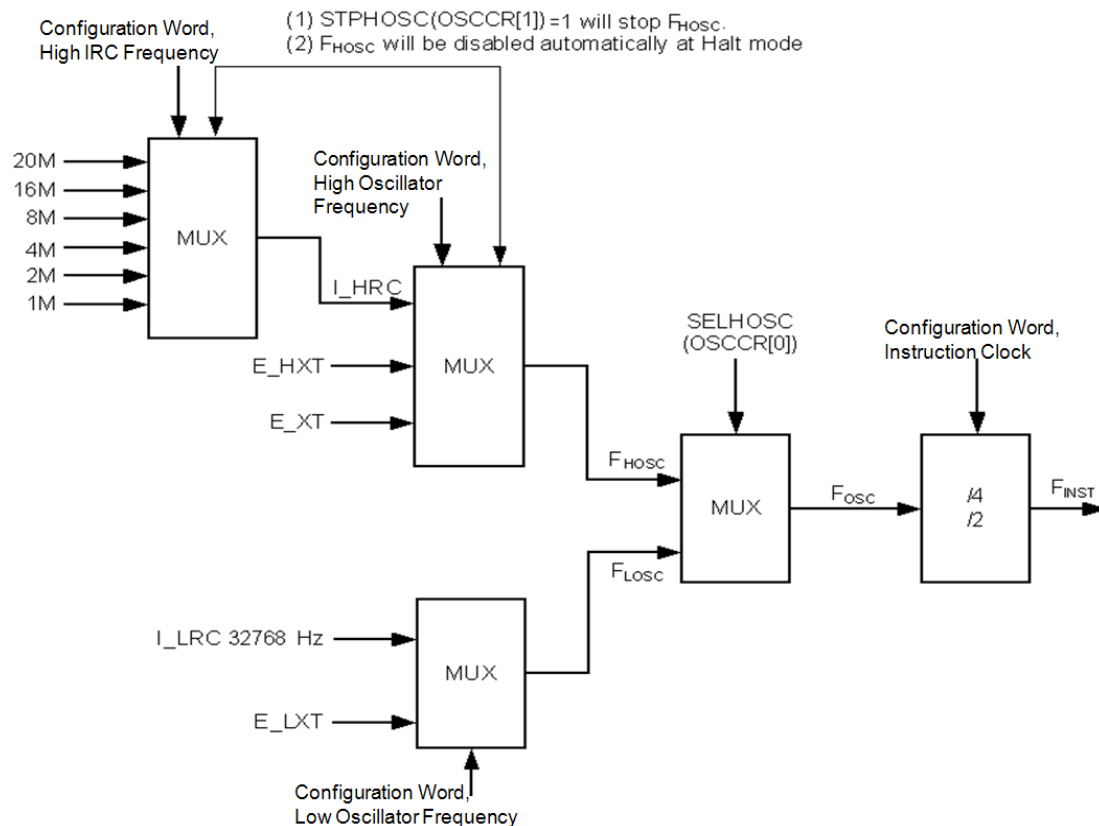
图 34 NY8B062F1 振荡配置结构图
