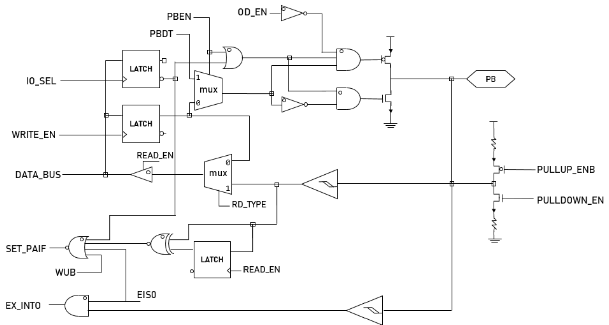
图 10 PB0 引脚结构框图
