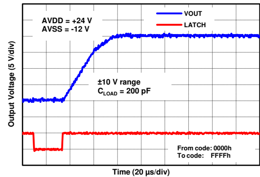
图 7-34. BP10V Rising
