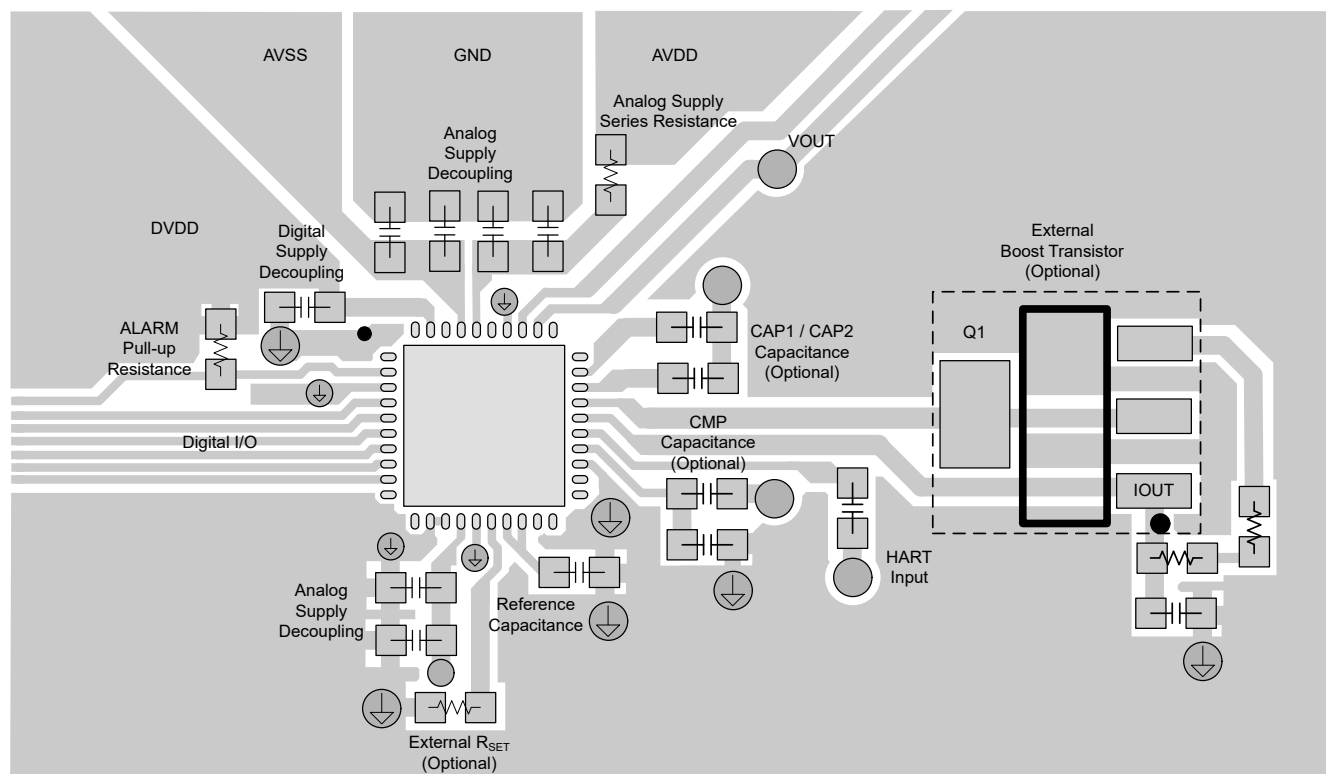
图 11-1. DACx760 Layout Example
