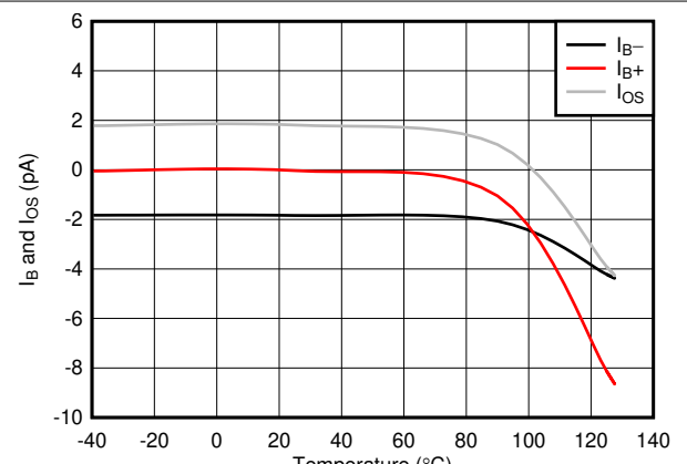
图 7-6. I_B 和 I_{OS} 与温度间的关系
