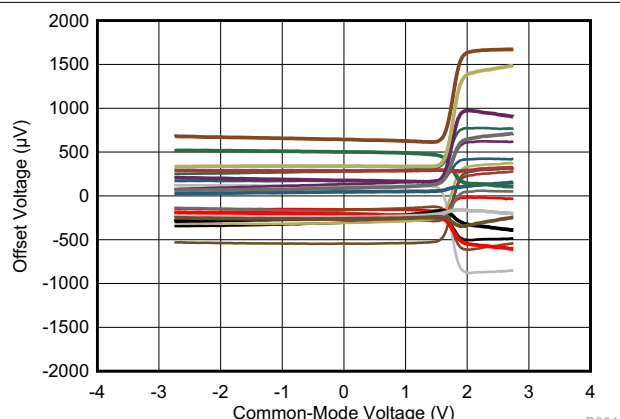
图 7-4. 失调电压与共模间的关系
