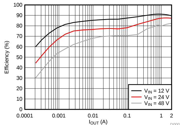
效率与输出电流间的关系 ( V_{OUT} = 5V , f_{sw} = 500kHz )
