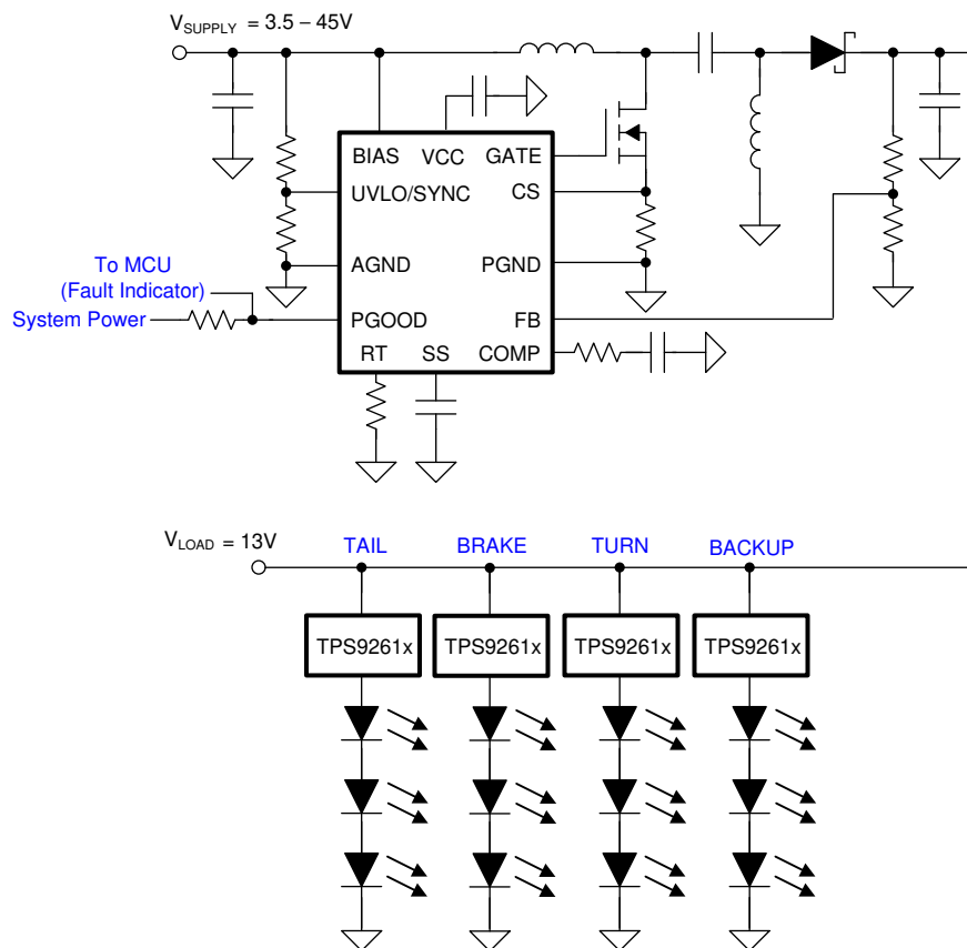
图 10-14. 两级汽车尾灯 LED 驱动器
