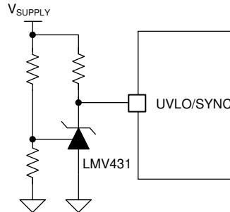
图 9-16. 反相 UVLO
