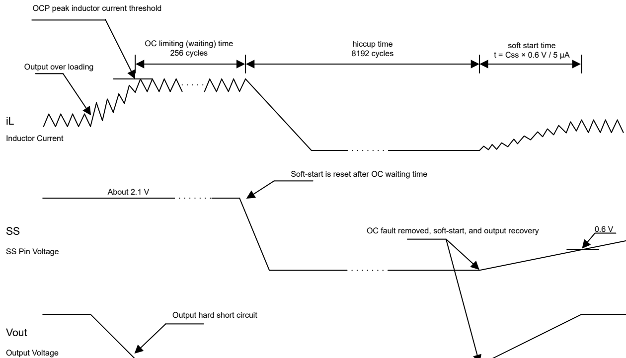
图 7-11. Overcurrent Protection
