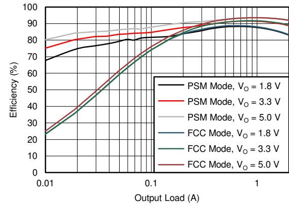
图 6-2. BUCK 2 Efficiency
