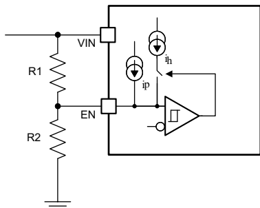
图 7-3. Adjustable VIN Undervoltage Lockout
