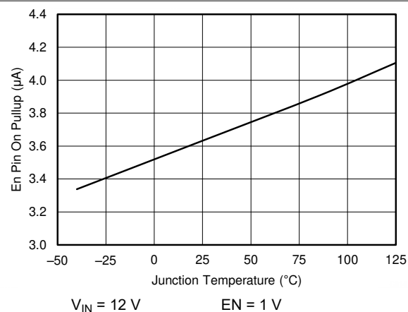
图 6-12. EN Pin Pull-Up Current vs Temperature, EN=1.0V
