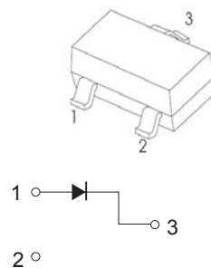
SOT-23
