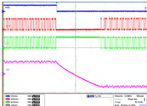
图 8-2. DRV8842 Current Regulation
