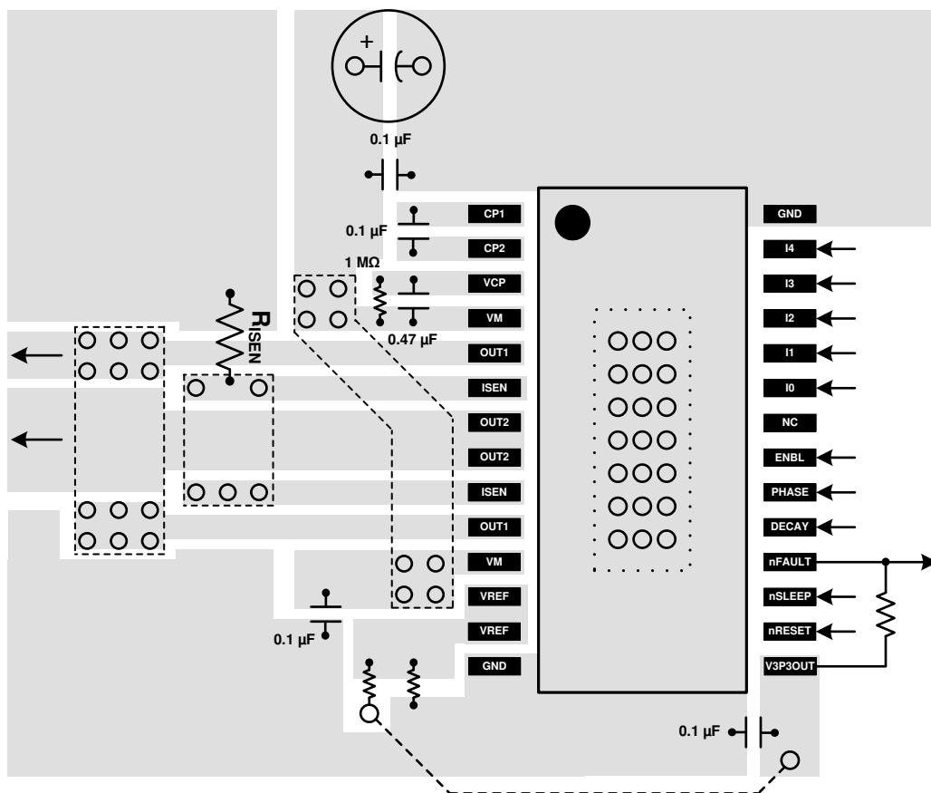
图 10-1. Example Layout
