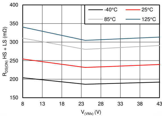
图 6-3. R_{DS(ON)} vs V_{(VMx)}
