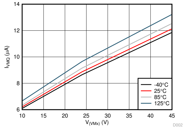
图 6-2. I_{VMxQ} vs V_{(VMx)}
