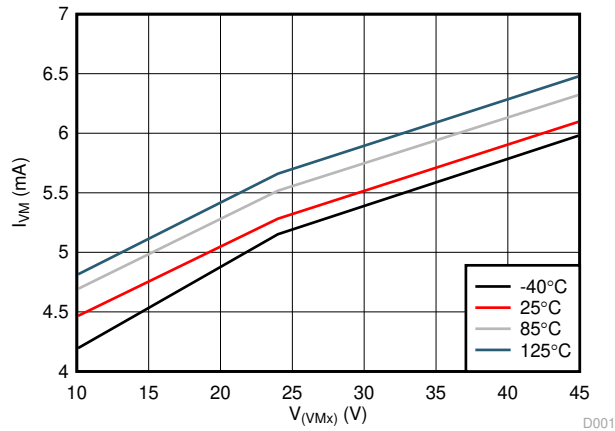
图 6-1. I_{VMx} vs V_{(VMx)}
