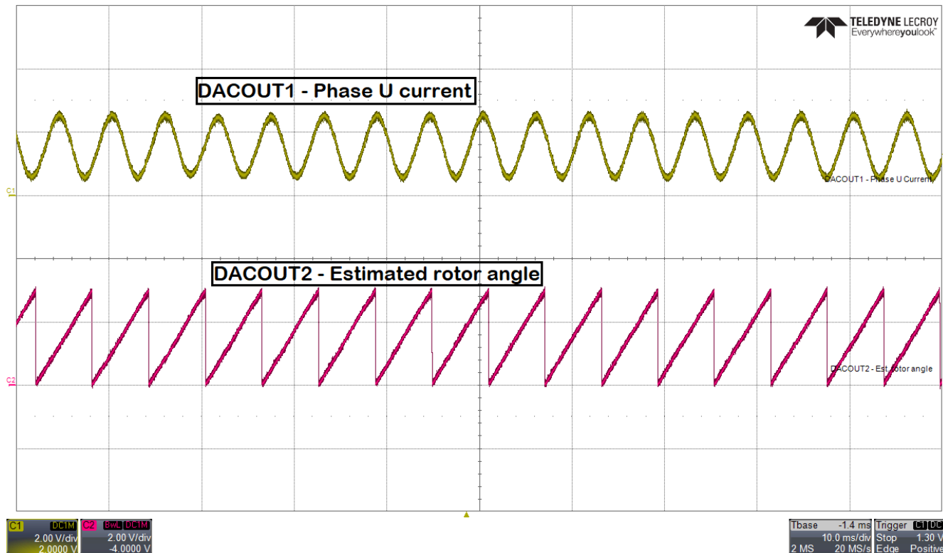
图 9-10. DACOUT1 和 DACOUT2
