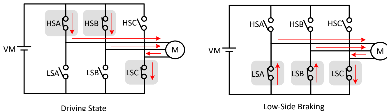
图 6-46. 低侧制动
