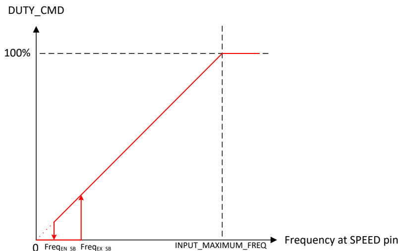
图 6-19. 频率模式速度控制
