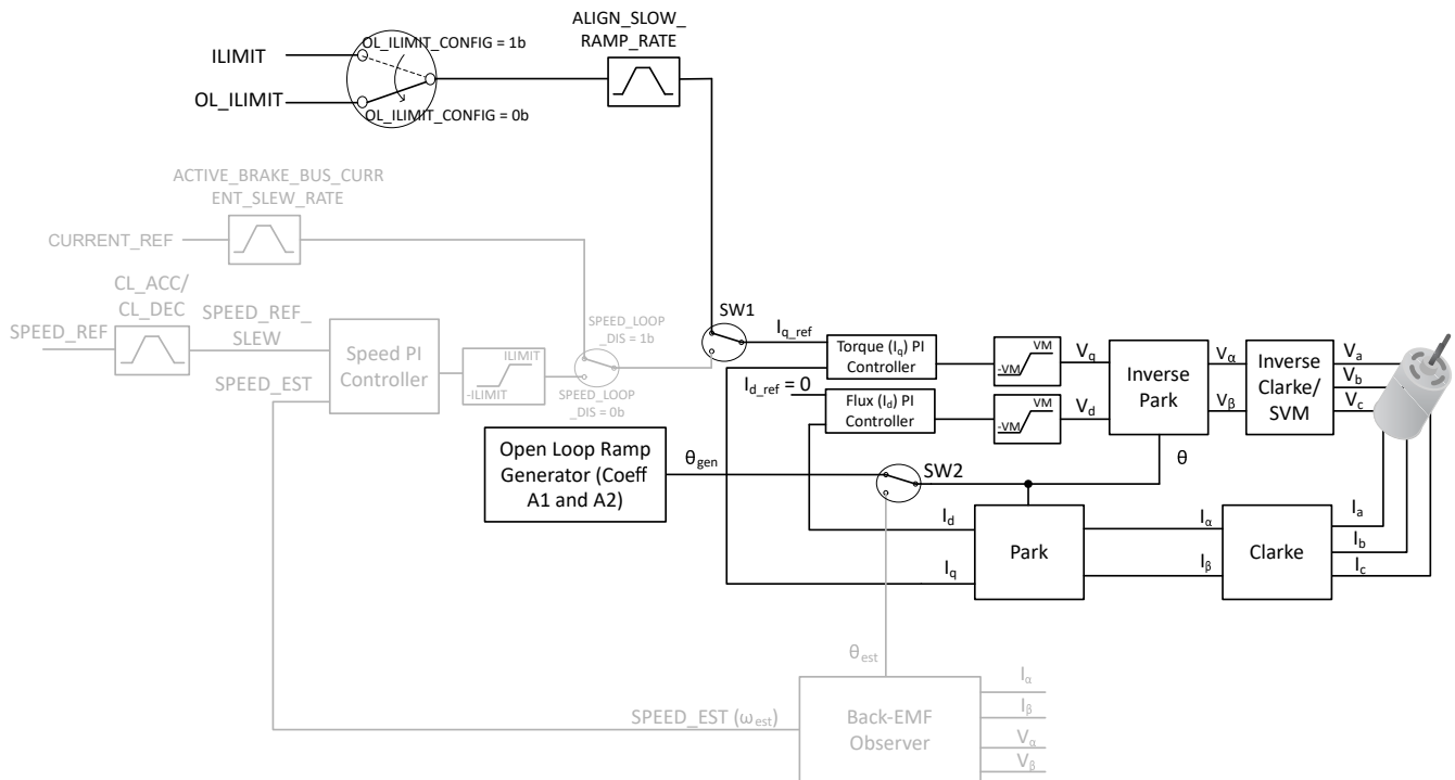
图 6-31. 开环
