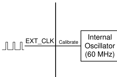
图 6-54. 外部时钟基准
