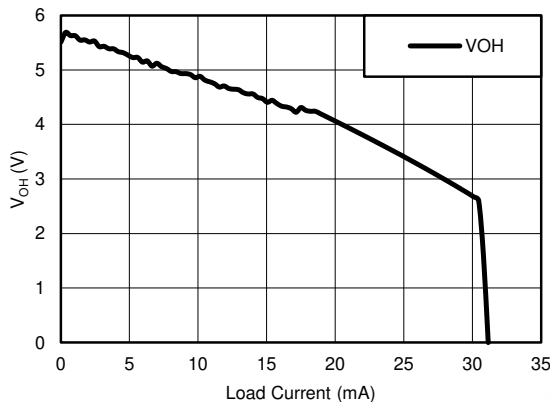
图 5-1. DOUT VOH vs Load Current
