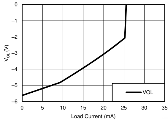
图 5-2. DOUT VOL vs Load Current
