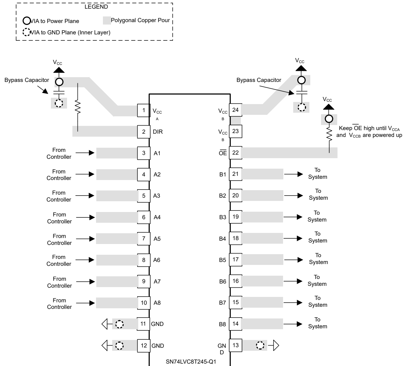
图 11-1. SN74LVC8T245-Q1 Layout
