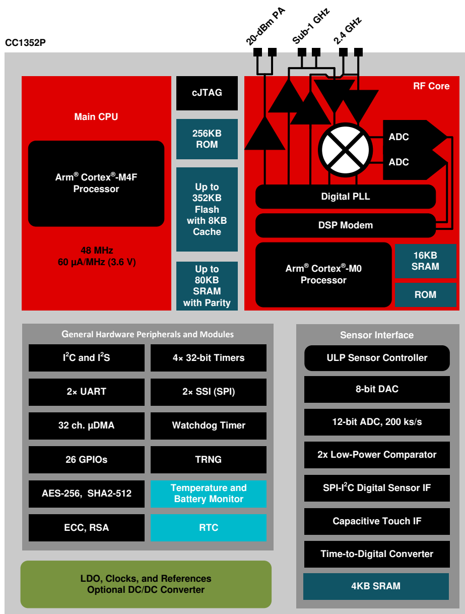
图 4-1. CC1352P Block Diagram
