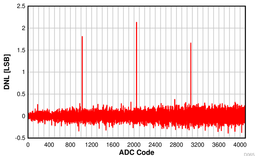
图 8-61. DNL vs. ADC Code
