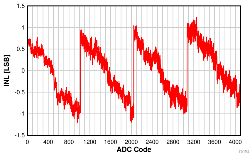
图 8-60. INL vs. ADC Code
