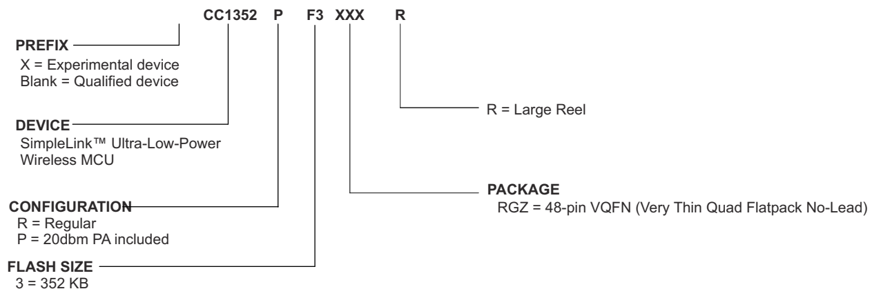
图 11-1. Device Nomenclature
