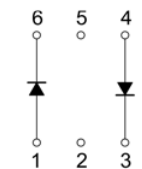
BAT54DW
