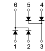
BAT54CDW
