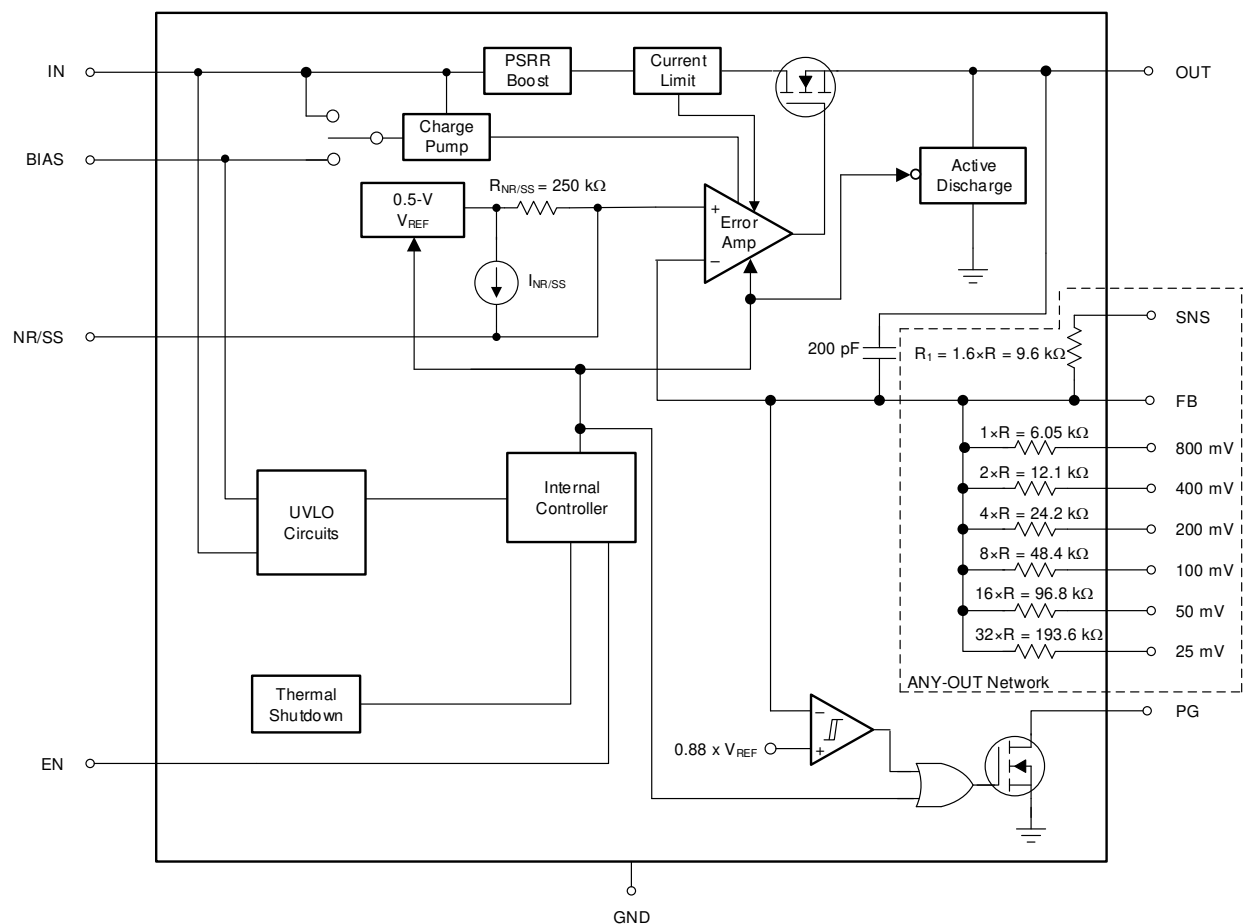
图 7-2. TPS7A8401A Block Diagram
