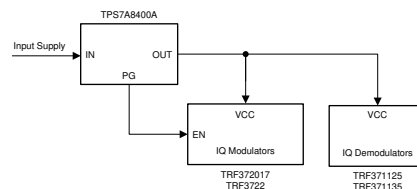
典型应用图
