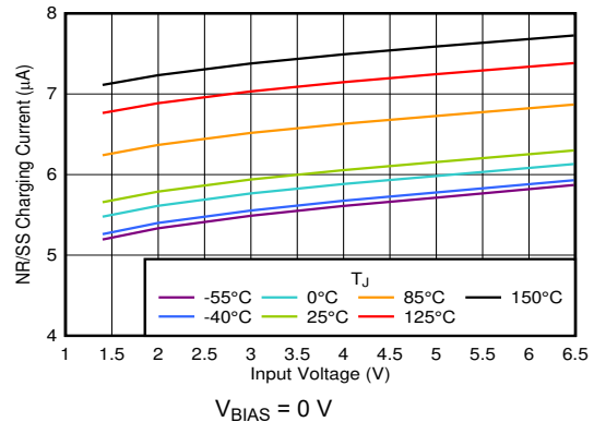
图 6-82. I_{NR/SS} Current vs V_{IN}
