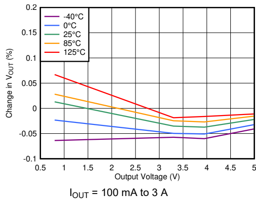
图 6-25. Load Regulation vs V_{OUT}
