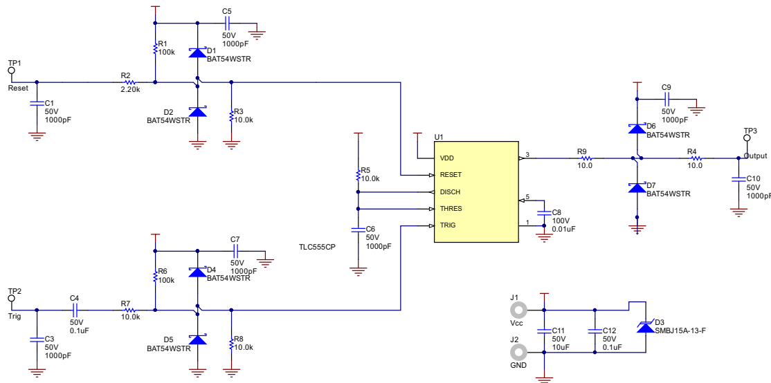
图 7-10. ESD Test Schematic
