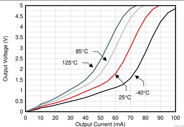
图 6-15. 输出电压摆幅与输出电流 (灌电流) 间的关系
