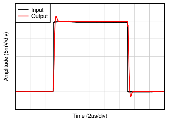
图 6-33. 正过载恢复
