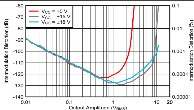
图 5-38. 互调失真与振幅间的关系
